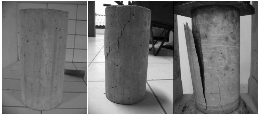
7 hari Beton Normal 240 KN
