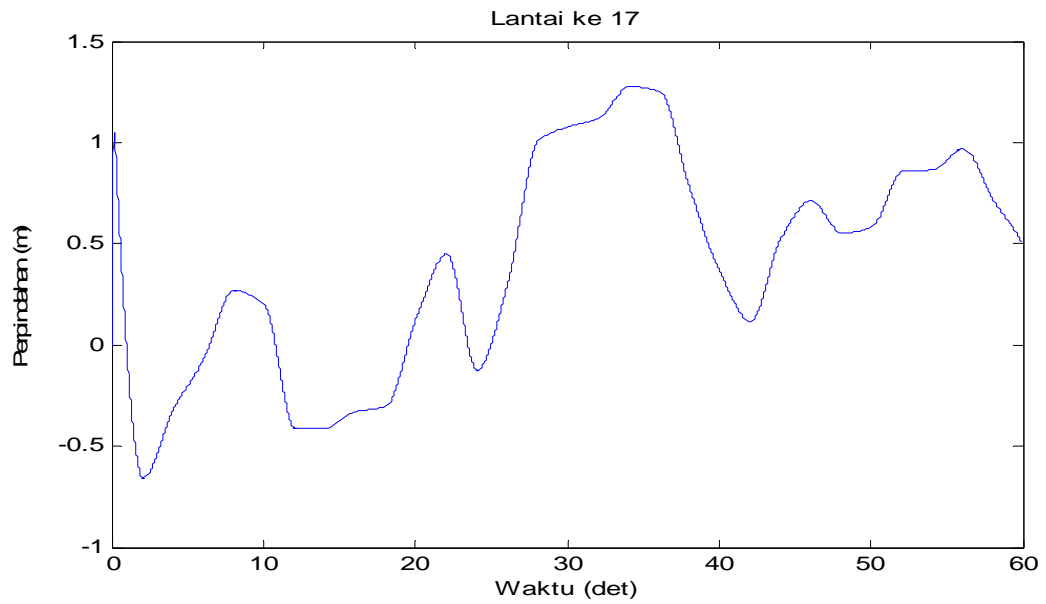
Gambar 4.108 Perpindahan di lantai 17 akibat beban gempa Flores dan Angin
