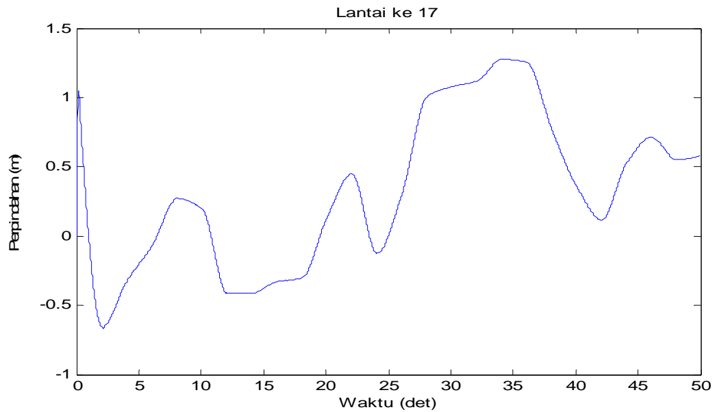
Gambar 4.88 Perpindahan di lantai 17 akibat beban gempa El-Centro dan Angin
