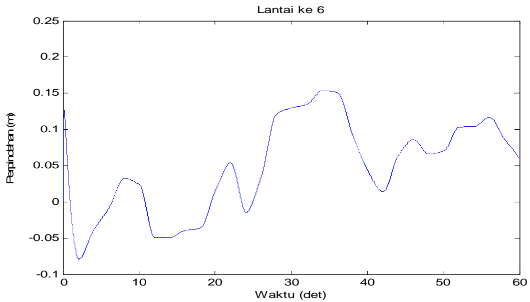
Gambar 4.97 Perpindahan di lantai 6 akibat beban gempa Flores dan Angin
