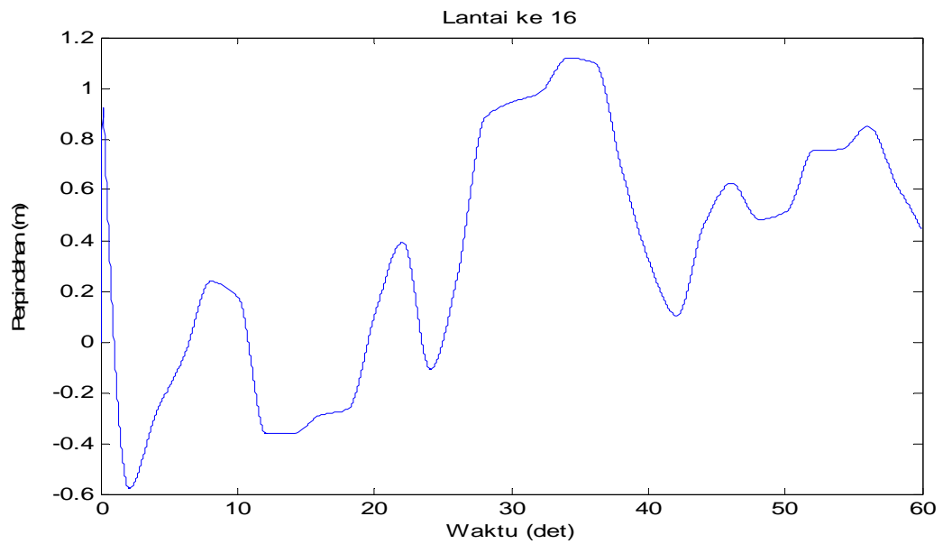
Gambar 4.107 Perpindahan di lantai 16 akibat beban gempa Flores dan Angin
