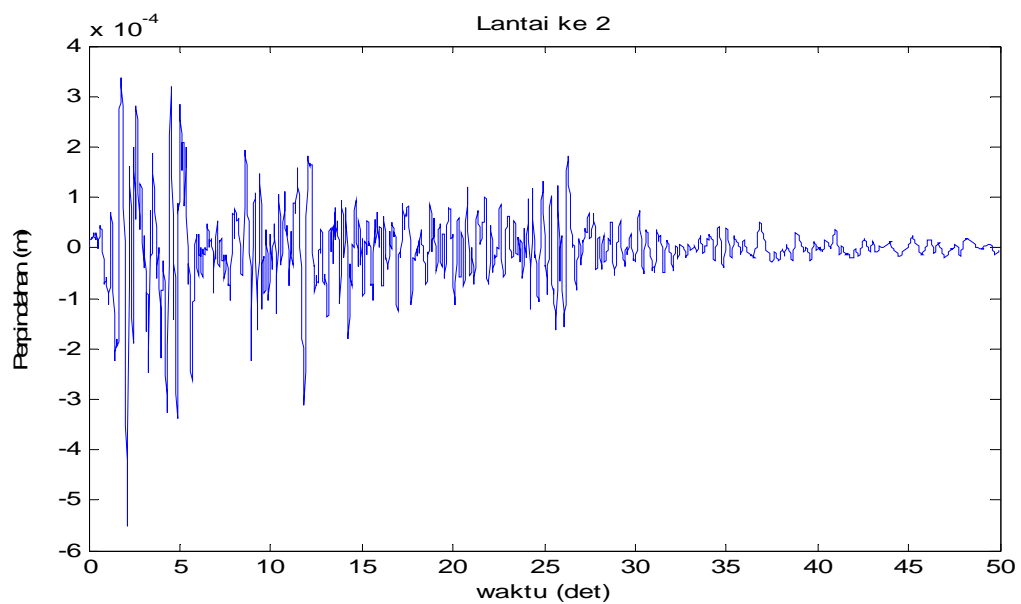
Gambar 4.13 Perpindahan di lantai 2 akibat beban gempa El-Centro
