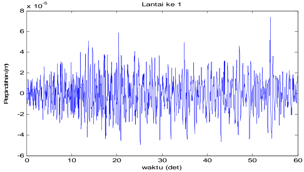
Gambar 4.32 Perpindahan di lantai 1 akibat beban gempa Flores
