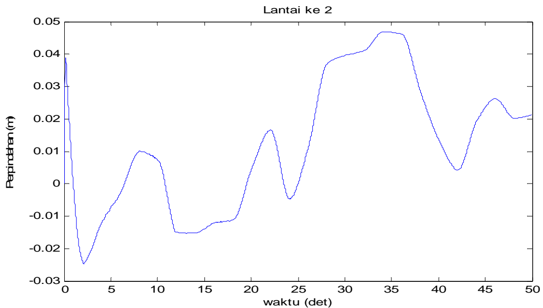
Gambar 4.73 Perpindahan di lantai 2 akibat beban gempa El-Centro dan Angin
