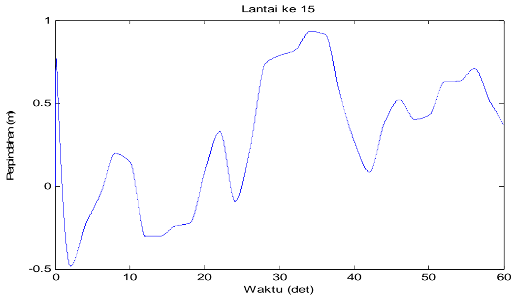
Gambar 4.66 Perpindahan di lantai 15 akibat beban Angin
