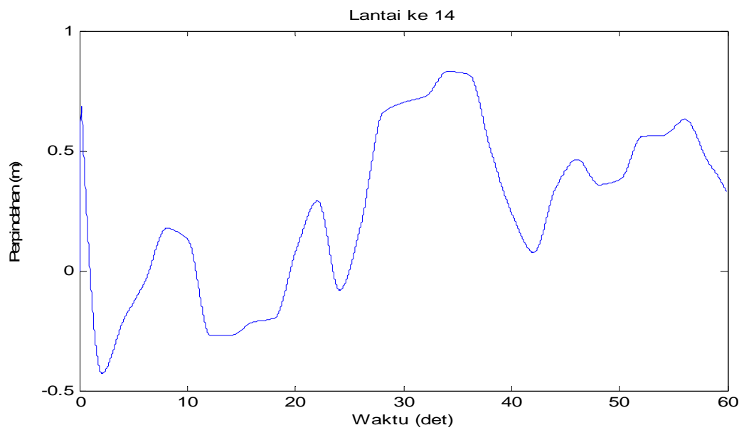
Gambar 4.65 Perpindahan di lantai 14 akibat beban Angin
