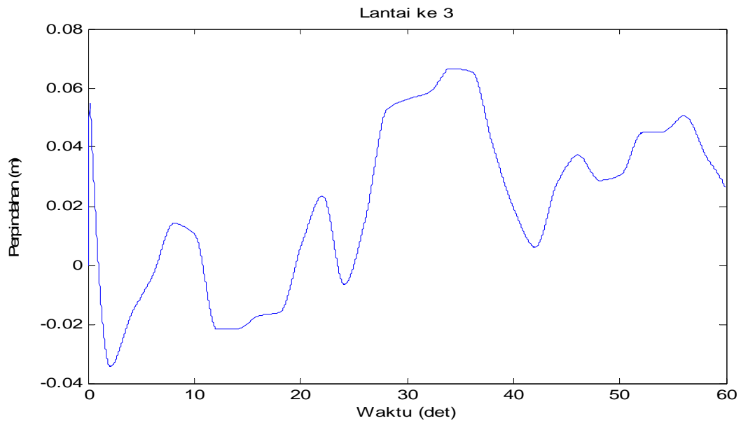
Gambar 4.54 Perpindahan di lantai 3 akibat beban Angin
