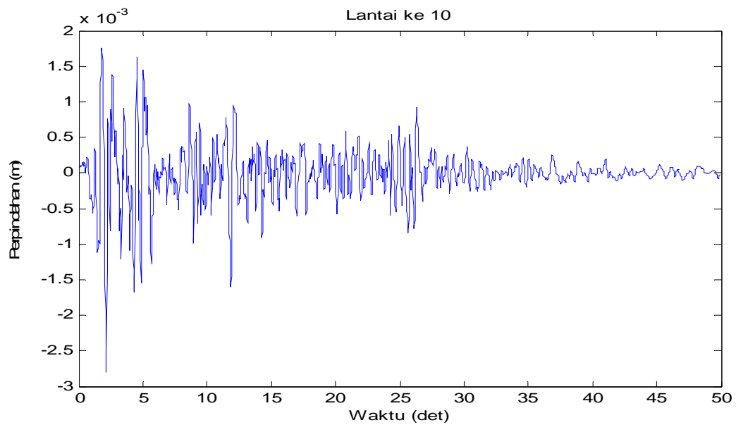
Gambar 4.21 Perpindahan di lantai 10 akibat beban gempa El-Centro
