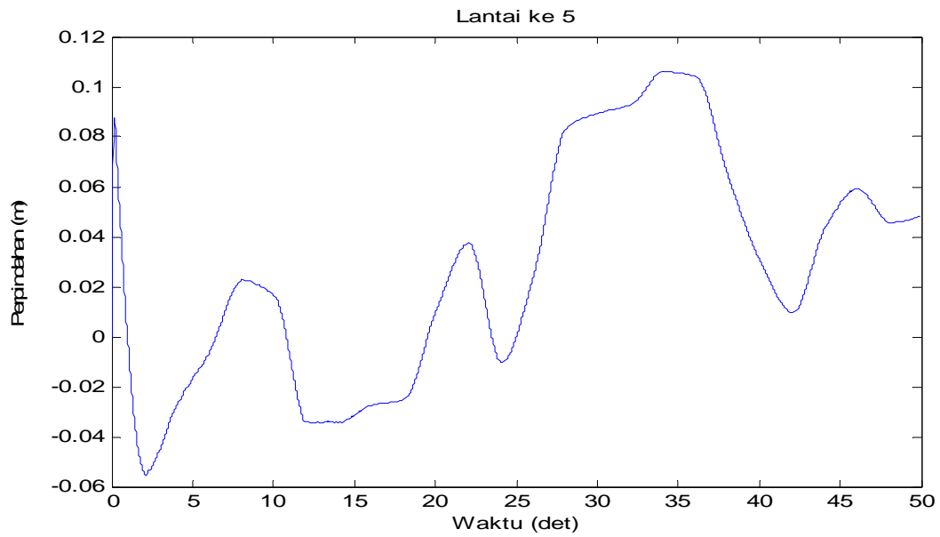
Gambar 4.76 Perpindahan di lantai 5 akibat beban gempa El-Centro dan Angin
