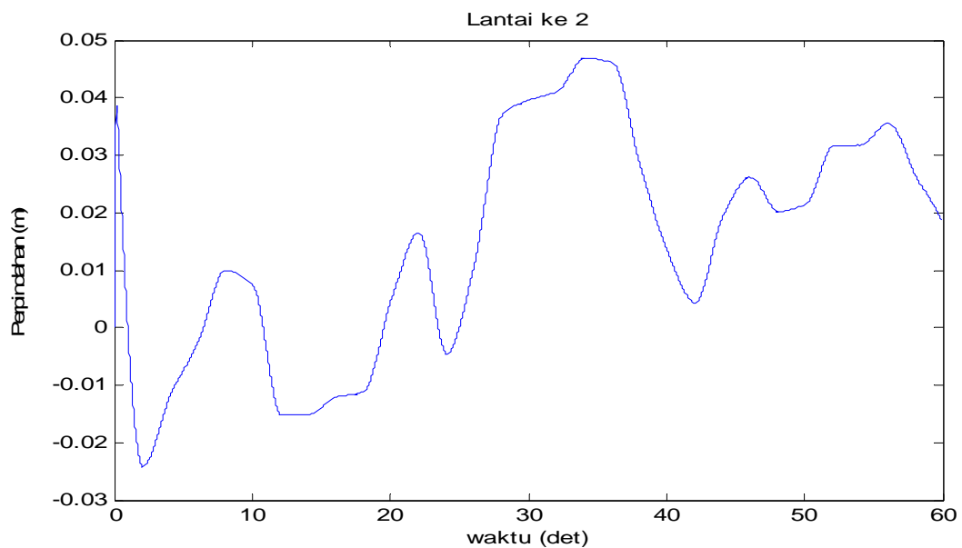
Gambar 4.93 Perpindahan di lantai 2 akibat beban gempa Flores dan Angin
