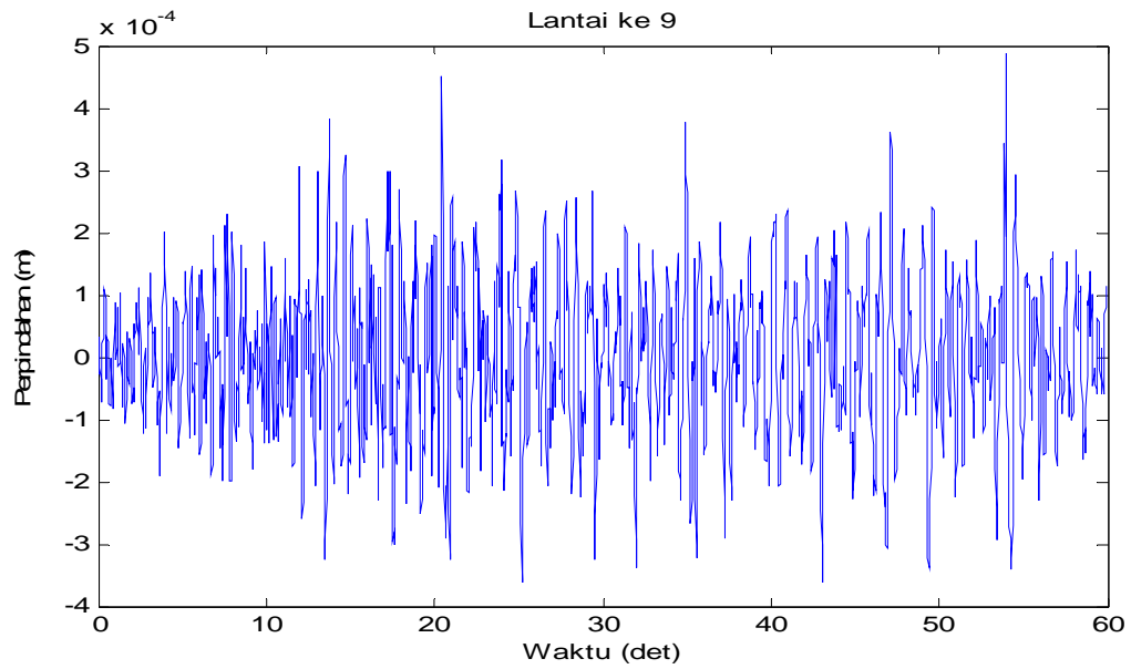
Gambar 4.40 Perpindahan di lantai 9 akibat beban gempa Flores
