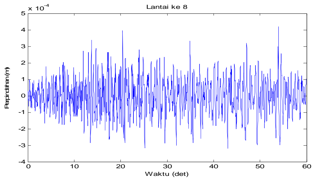
Gambar 4.39 Perpindahan di lantai 8 akibat beban gempa Flores
