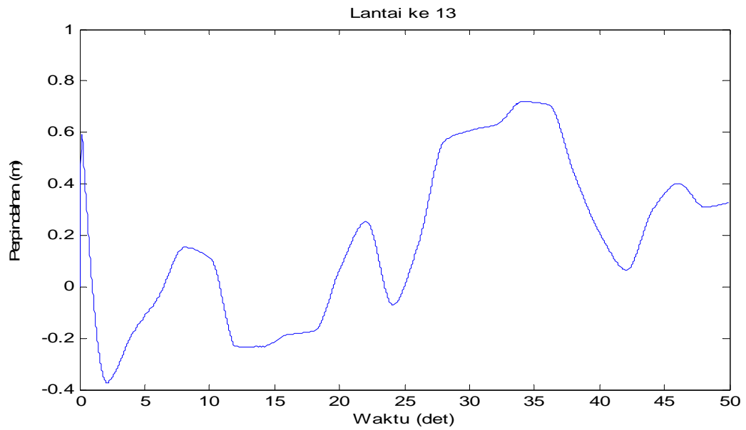
Gambar 4.84 Perpindahan di lantai 13 akibat beban gempa El-Centro dan Angin
