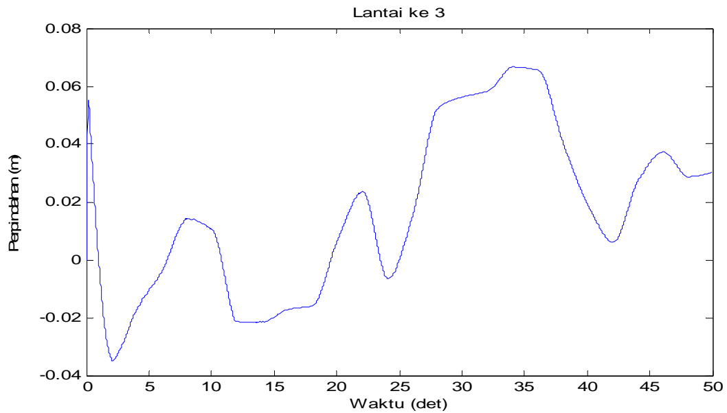
Gambar 4.74 Perpindahan di lantai 3 akibat beban gempa El-Centro dan Angin
