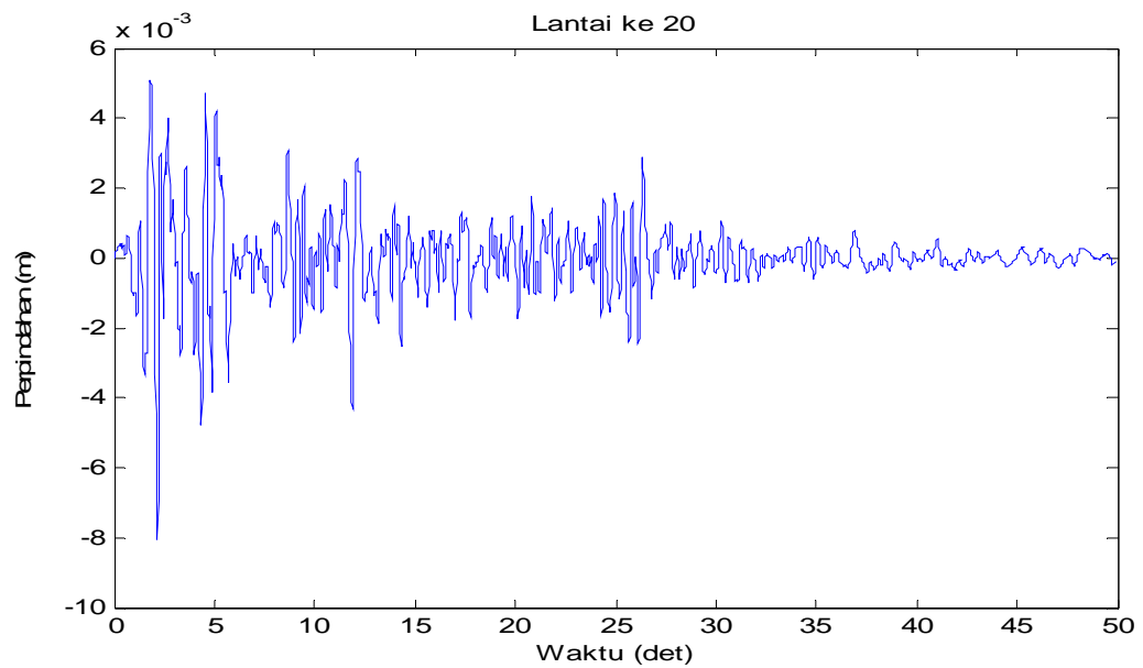
Gambar 4.31 Perpindahan di lantai 20 akibat beban gempa El-Centro
