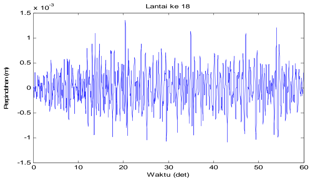
Gambar 4.49 Perpindahan di lantai 18 akibat beban gempa Flores
