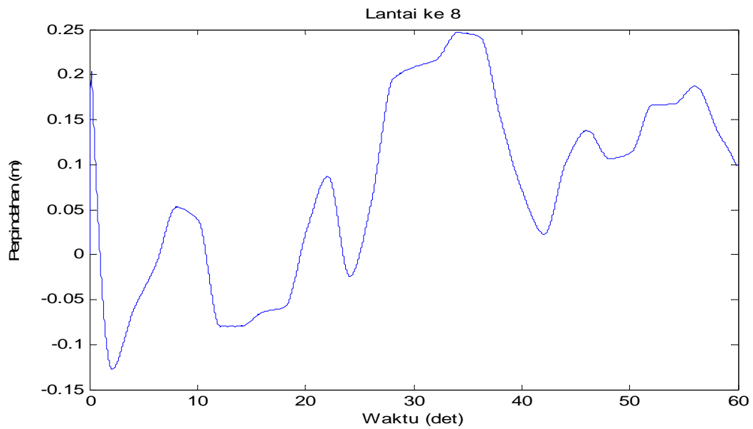
Gambar 4.99 Perpindahan di lantai 8 akibat beban gempa Flores dan Angin
