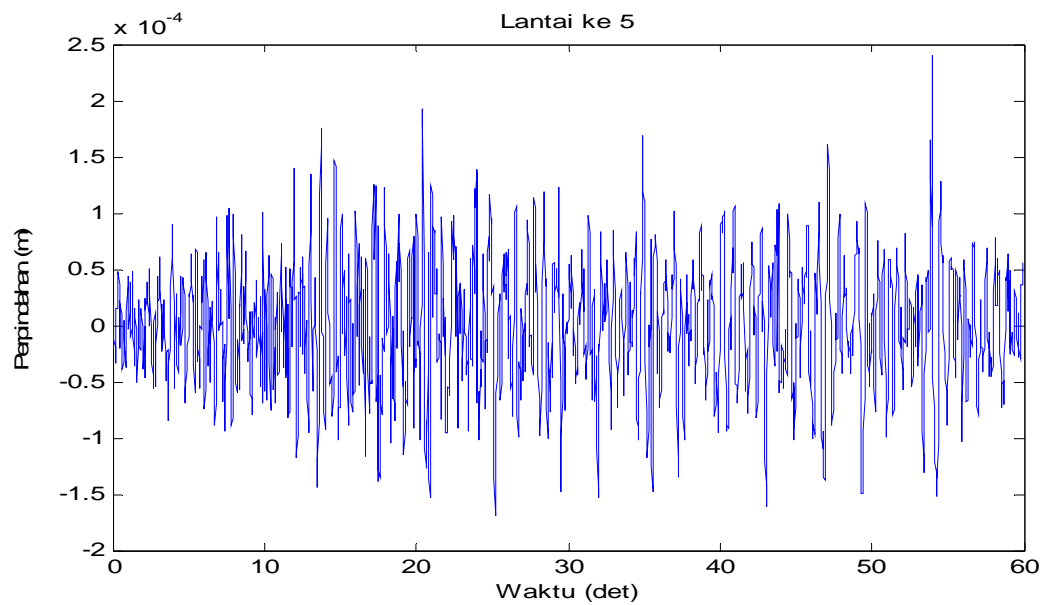
Gambar 4.36 Perpindahan di lantai 5 akibat beban gempa Flores
