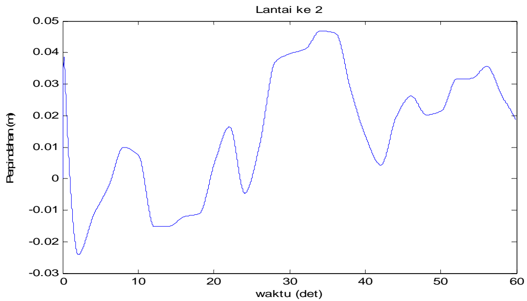
Gambar 4.53 Perpindahan di lantai 2 akibat beban Angin
