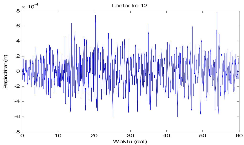
Gambar 4.43 Perpindahan di lantai 12 akibat beban gempa Flores
