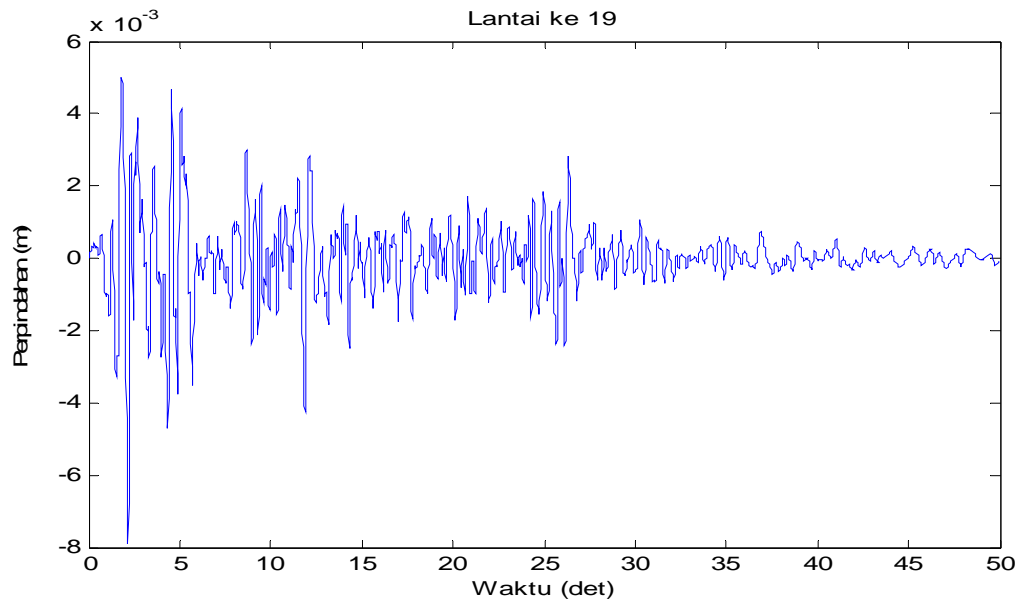
Gambar 4.30 Perpindahan di lantai 19 akibat beban gempa El-Centro
