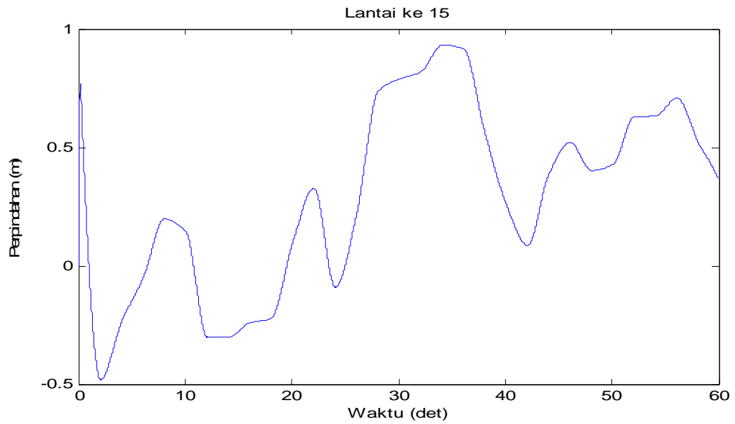
Gambar 4.106 Perpindahan di lantai 15 akibat beban gempa Flores dan Angin
