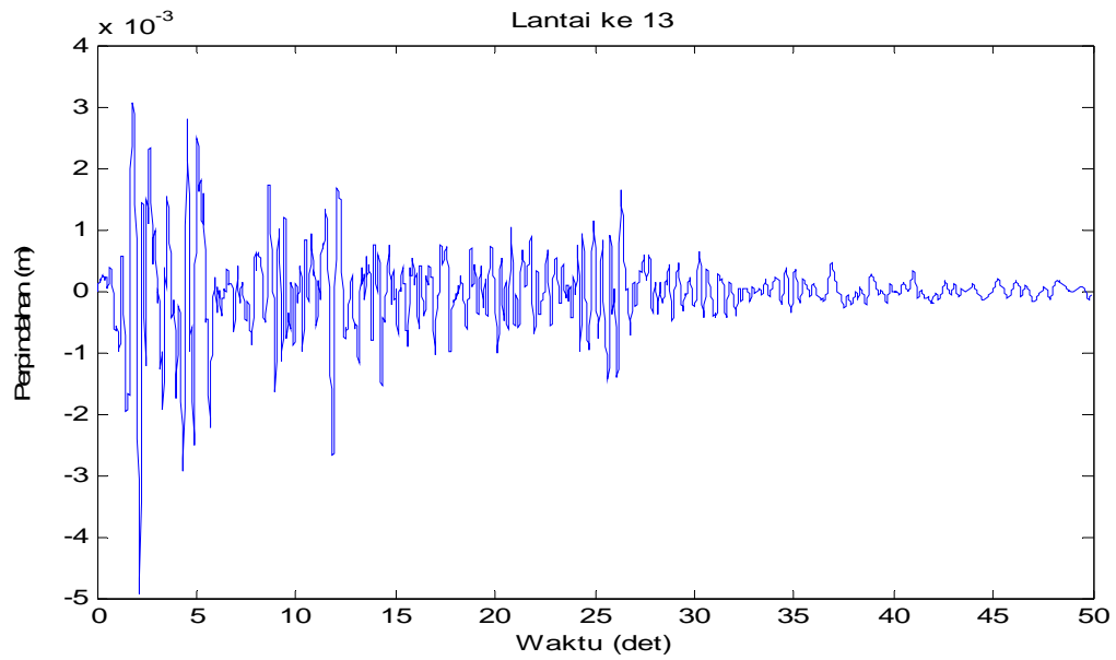
Gambar 4.24 Perpindahan di lantai 13 akibat beban gempa El-Centro
