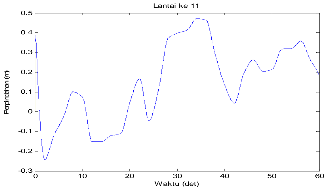
Gambar 4.102 Perpindahan di lantai 11 akibat beban gempa Flores dan Angin
