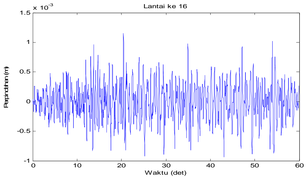
Gambar 4.47 Perpindahan di lantai 16 akibat beban gempa Flores
