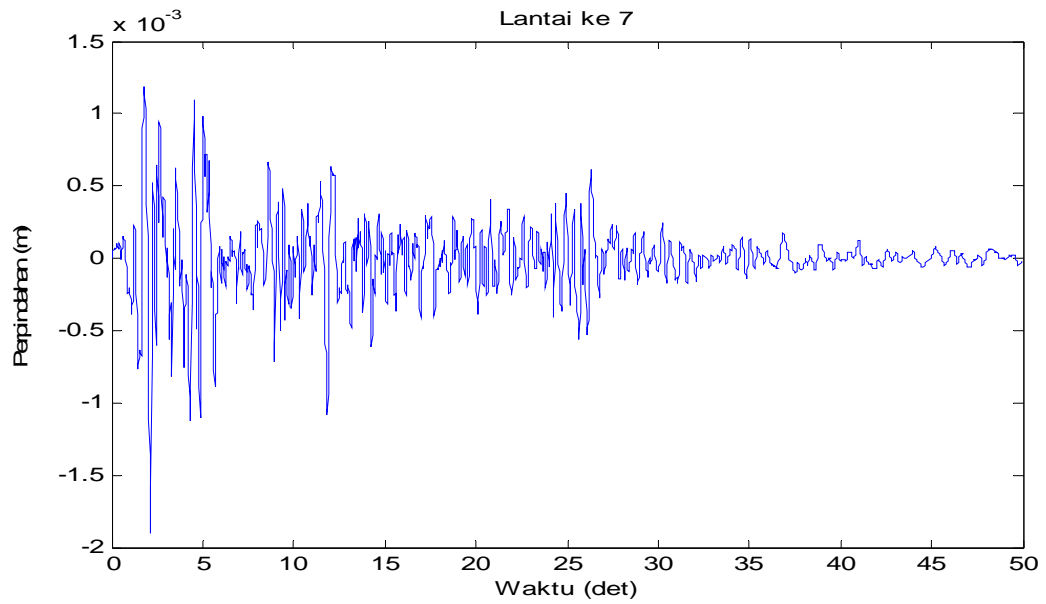
Gambar 4.18 Perpindahan di lantai 7 akibat beban gempa El-Centro
