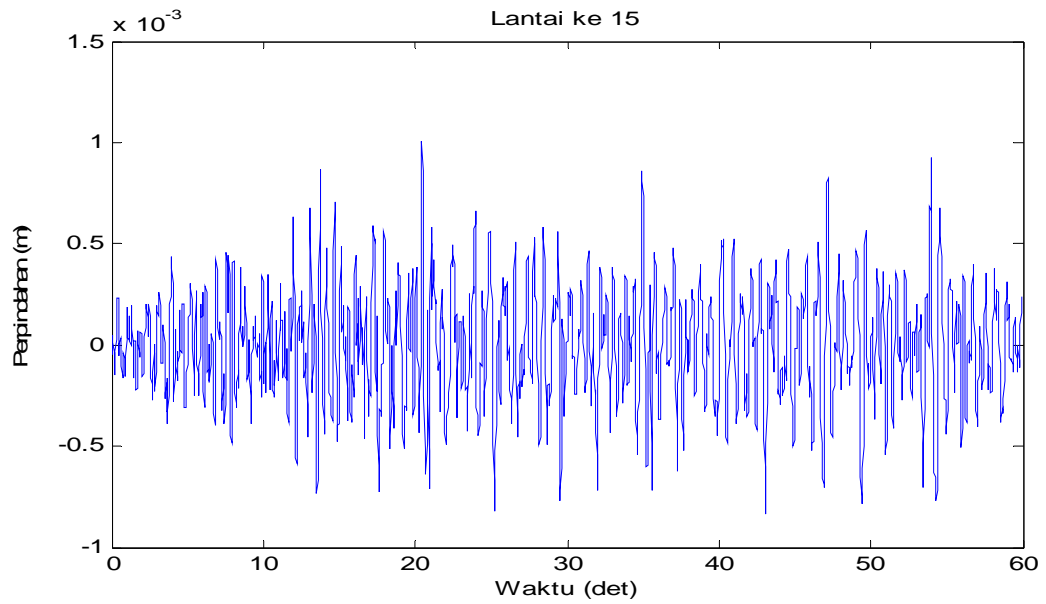
Gambar 4.46 Perpindahan di lantai 15 akibat beban gempa Flores
