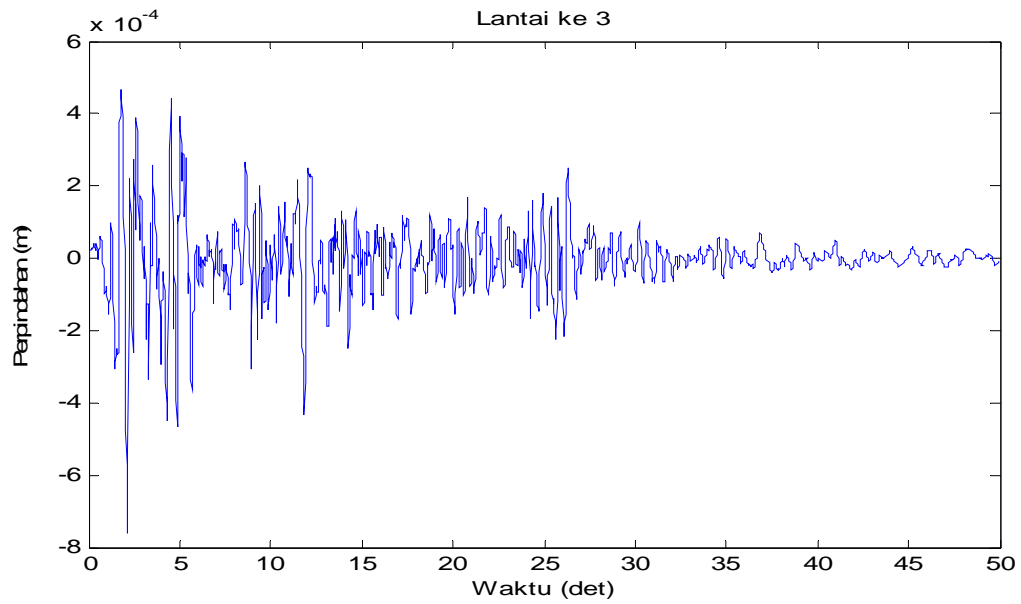
Gambar 4.14 Perpindahan di lantai 3 akibat beban gempa El-Centro
