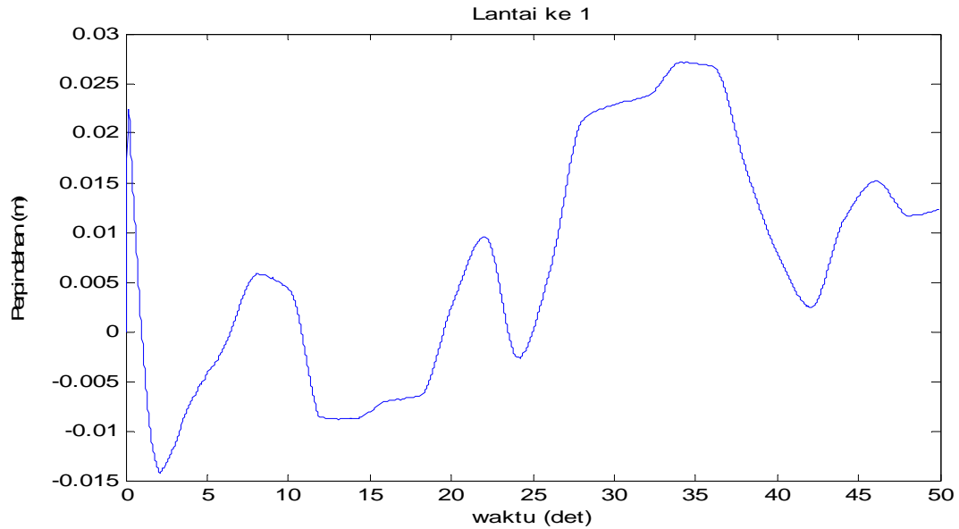
Gambar 4.72 Perpindahan di lantai 1 akibat beban gempa El-Centro dan Angin
