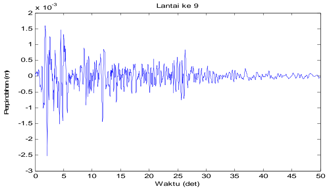
Gambar 4.20 Perpindahan di lantai 9 akibat beban gempa El-Centro
