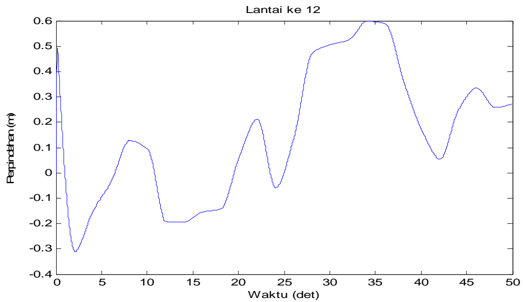
Gambar 4.83 Perpindahan di lantai 12 akibat beban gempa El-Centro dan Angin
