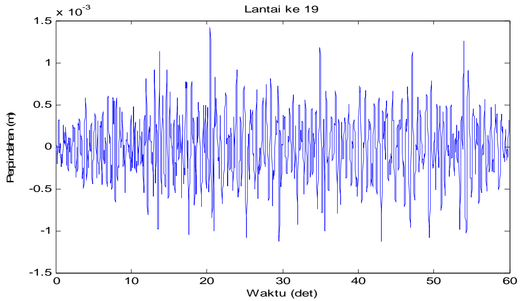
Gambar 4.50 Perpindahan di lantai 19 akibat beban gempa Flores
