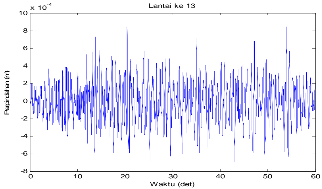
Gambar 4.44 Perpindahan di lantai 13 akibat beban gempa Flores
