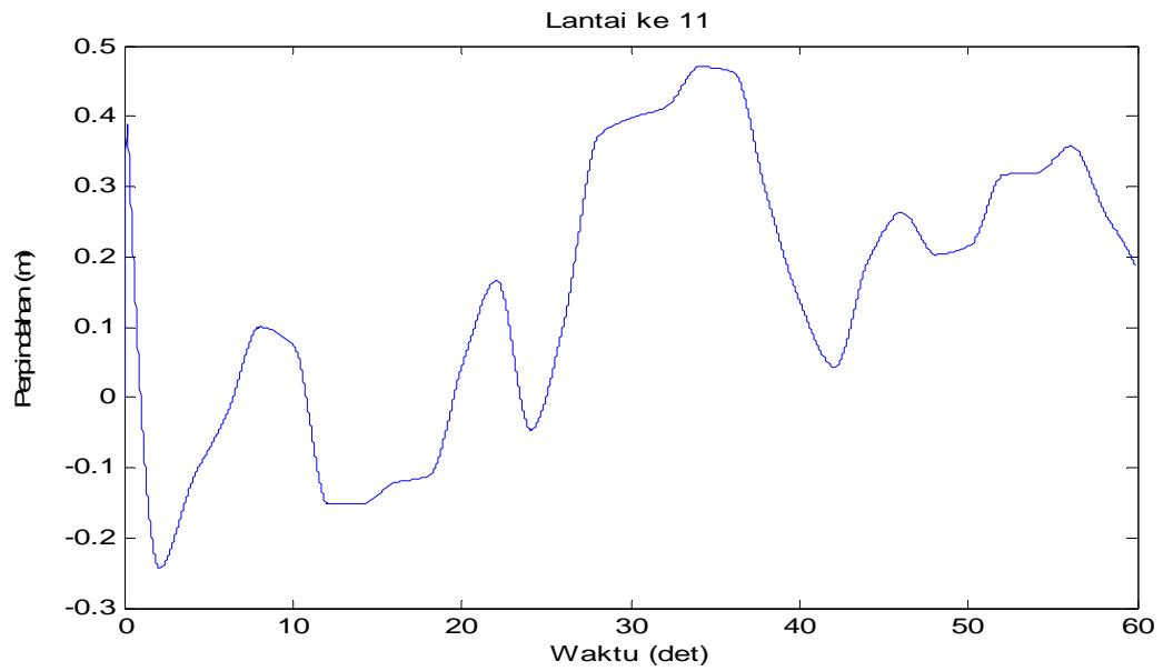
Gambar 4.62 Perpindahan di lantai 11 akibat beban Angin
