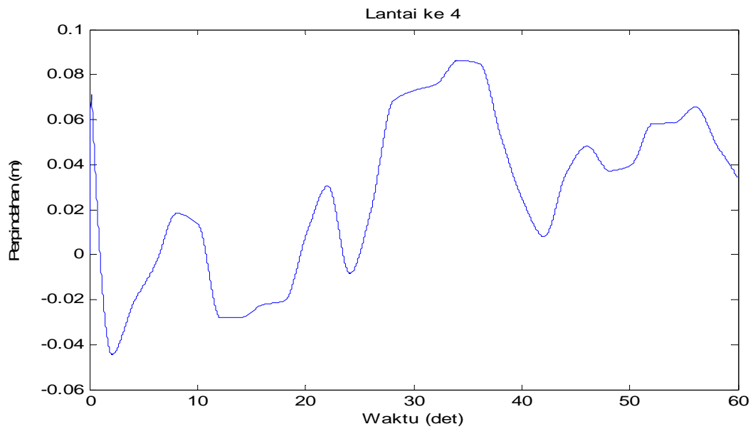
Gambar 4.55 Perpindahan di lantai 4 akibat beban Angin
