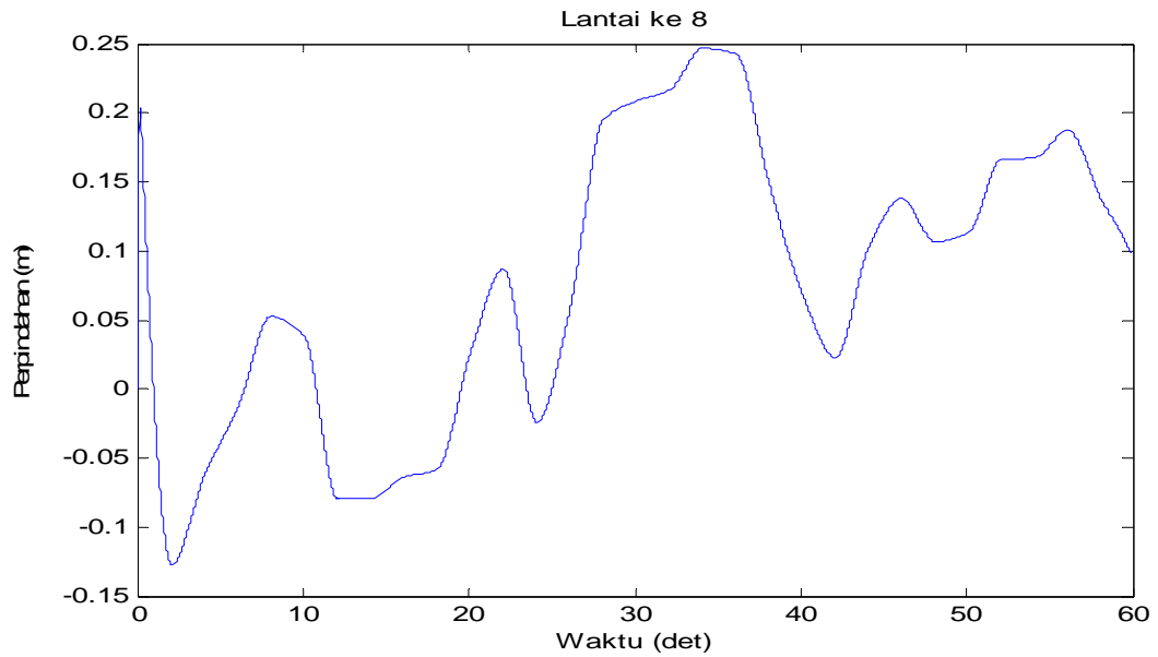
Gambar 4.59 Perpindahan di lantai 8 akibat beban Angin
