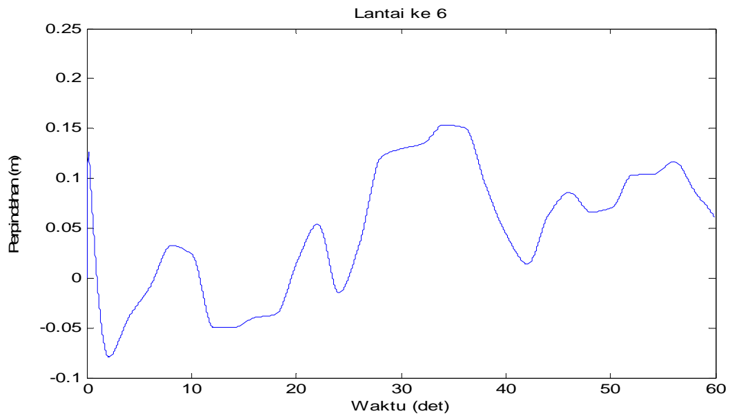
Gambar 4.57 Perpindahan di lantai 6 akibat beban Angin
