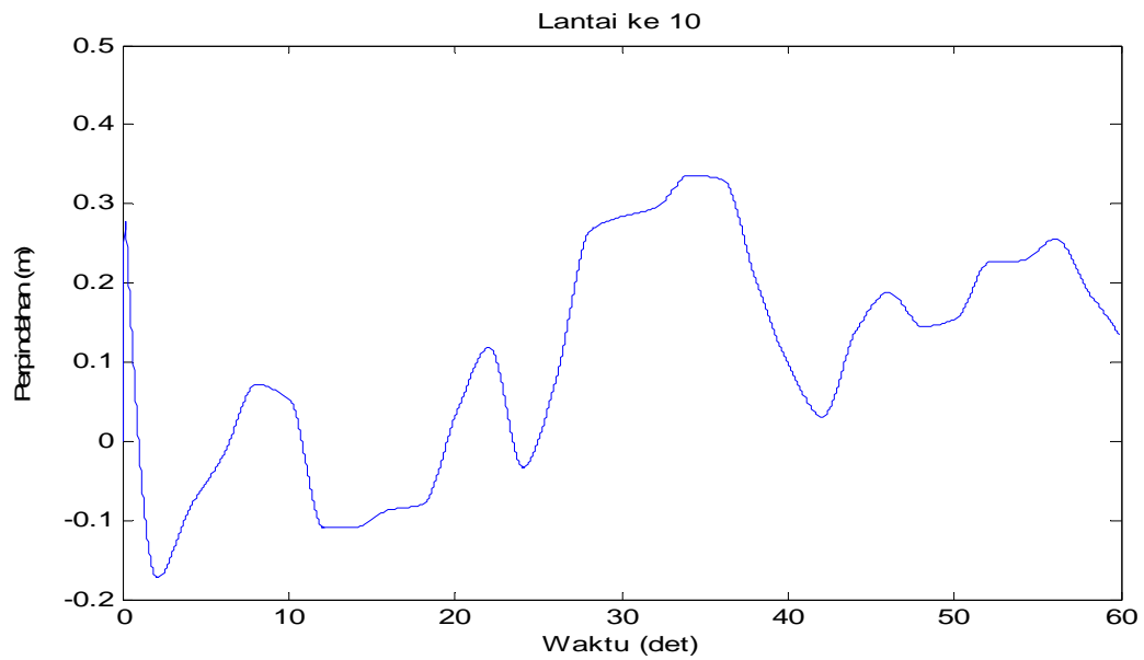
Gambar 4.61 Perpindahan di lantai 10 akibat beban Angin
