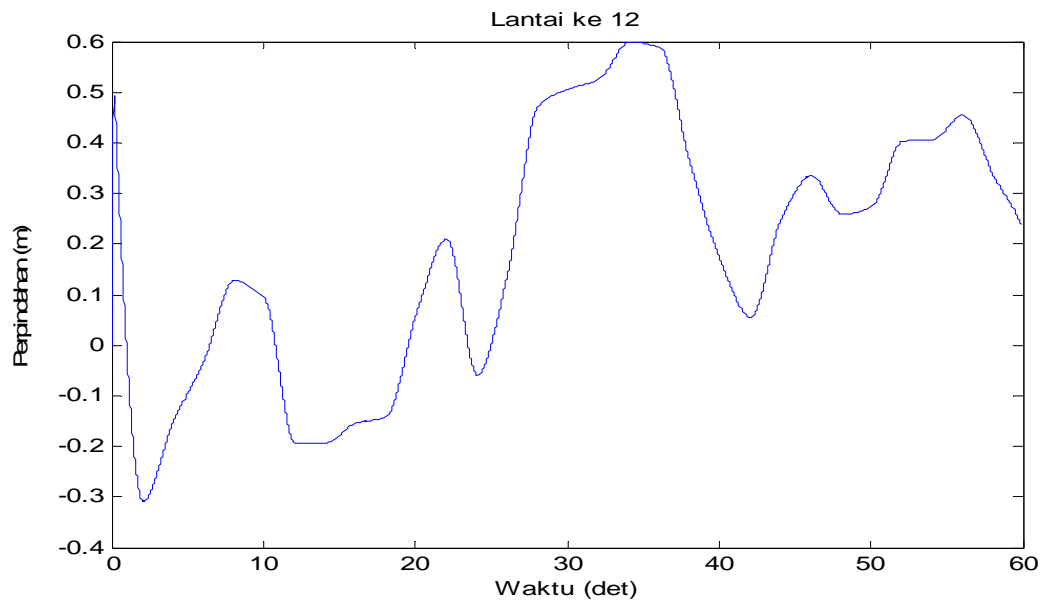
Gambar 4.103 Perpindahan di lantai 12 akibat beban gempa Flores dan Angin
