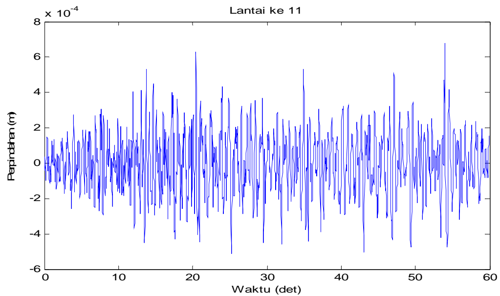
Gambar 4.42 Perpindahan di lantai 11 akibat beban gempa Flores
