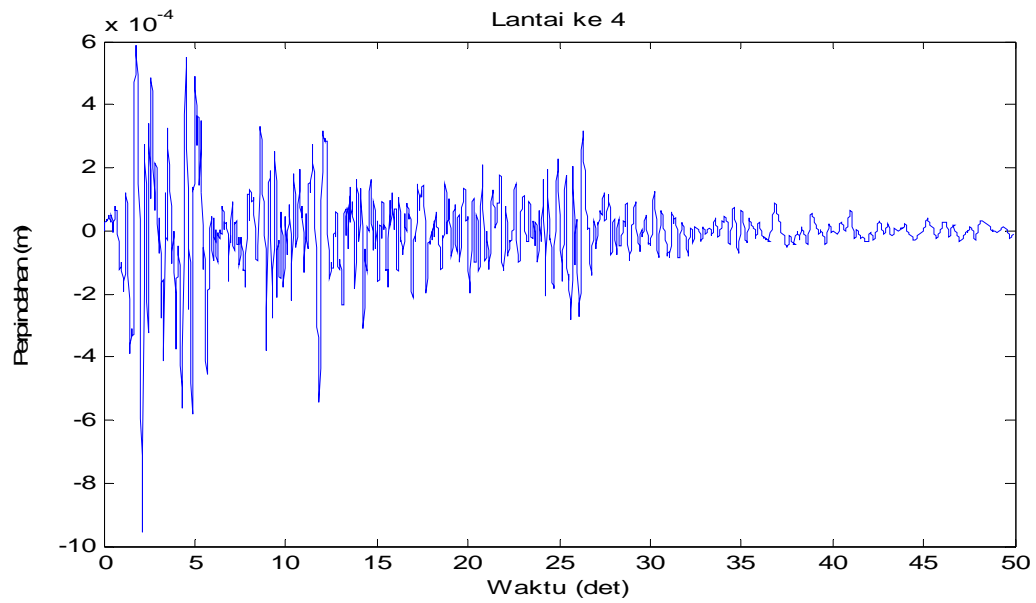
Gambar 4.15 Perpindahan di lantai 4 akibat beban gempa El-Centro
