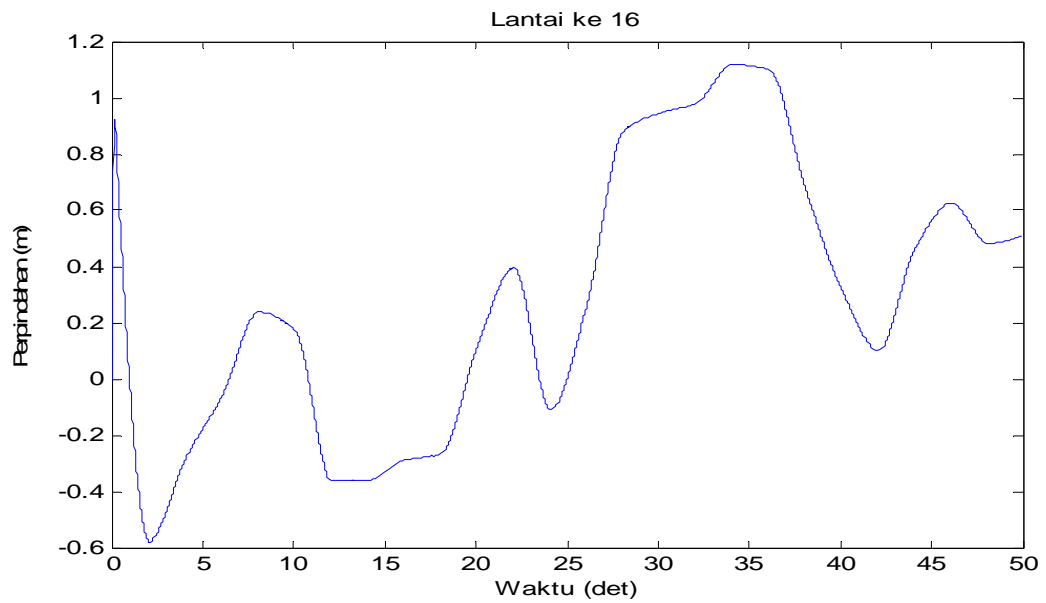
Gambar 4.87 Perpindahan di lantai 16 akibat beban gempa El-Centro dan Angin
