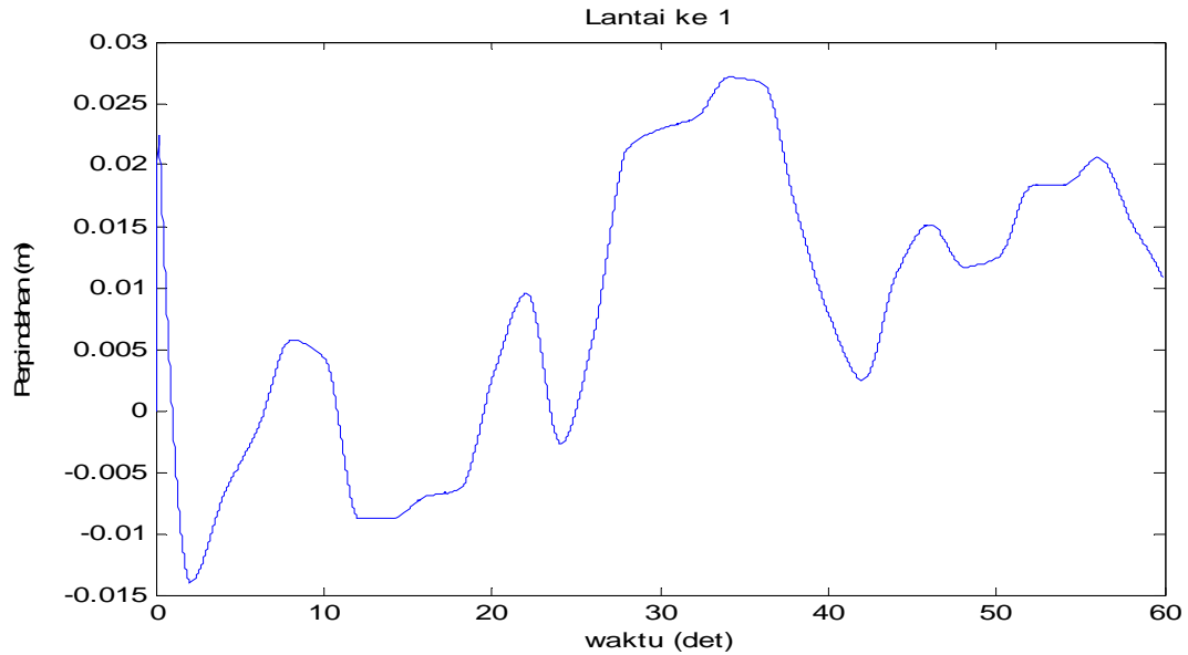
Gambar 4.92 Perpindahan di lantai 1 akibat beban gempa Flores dan Angin
