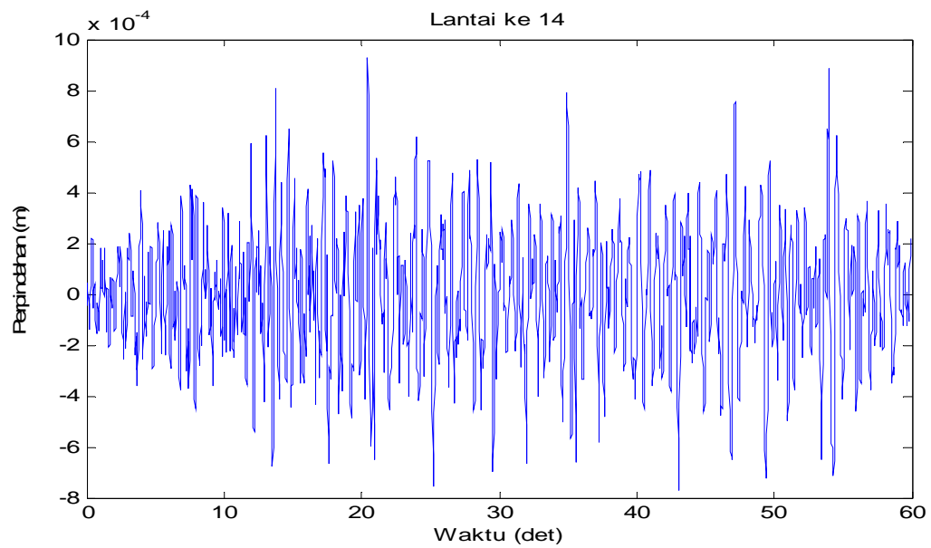
Gambar 4.45 Perpindahan di lantai 14 akibat beban gempa Flores
