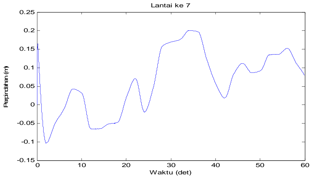
Gambar 4.98 Perpindahan di lantai 7 akibat beban gempa Flores dan Angin
