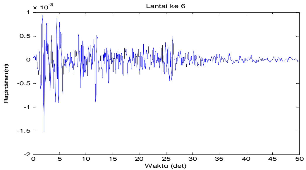
Gambar 4.17 Perpindahan di lantai 6 akibat beban gempa El-Centro
