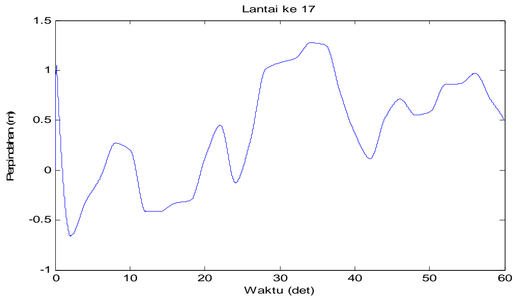
Gambar 4.68 Perpindahan di lantai 17 akibat beban Angin
