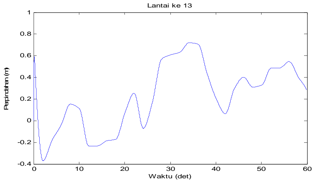
Gambar 4.64 Perpindahan di lantai 13 akibat beban Angin
