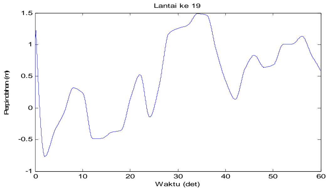
Gambar 4.70 Perpindahan di lantai 19 akibat beban Angin
