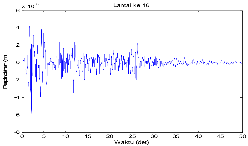
Gambar 4.27 Perpindahan di lantai 16 akibat beban gempa El-Centro
