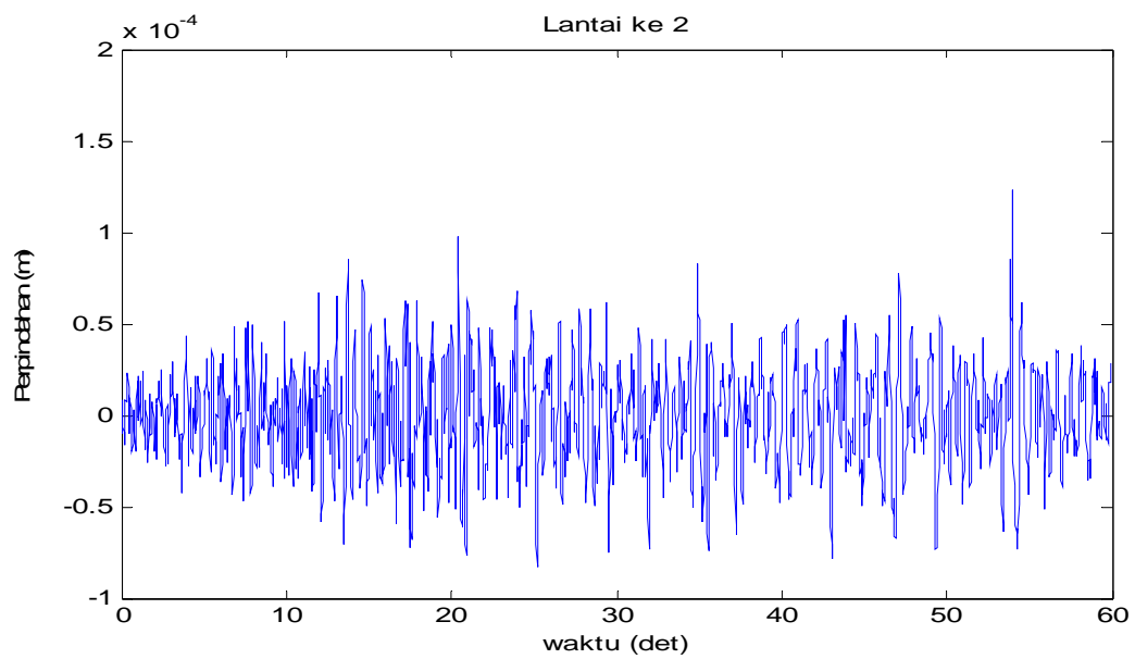
Gambar 4.33 Perpindahan di lantai 2 akibat beban gempa Flores
