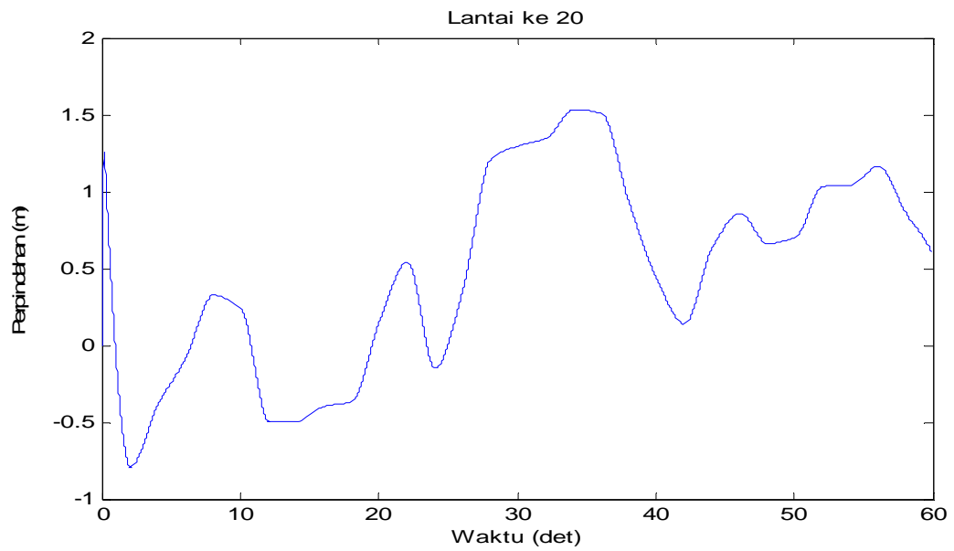
Gambar 4.71 Perpindahan di lantai 20 akibat beban Angin
