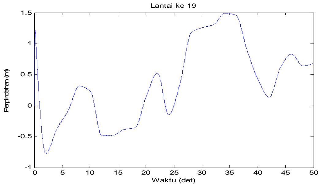
Gambar 4.90 Perpindahan di lantai 19 akibat beban gempa El-Centro dan Angin
