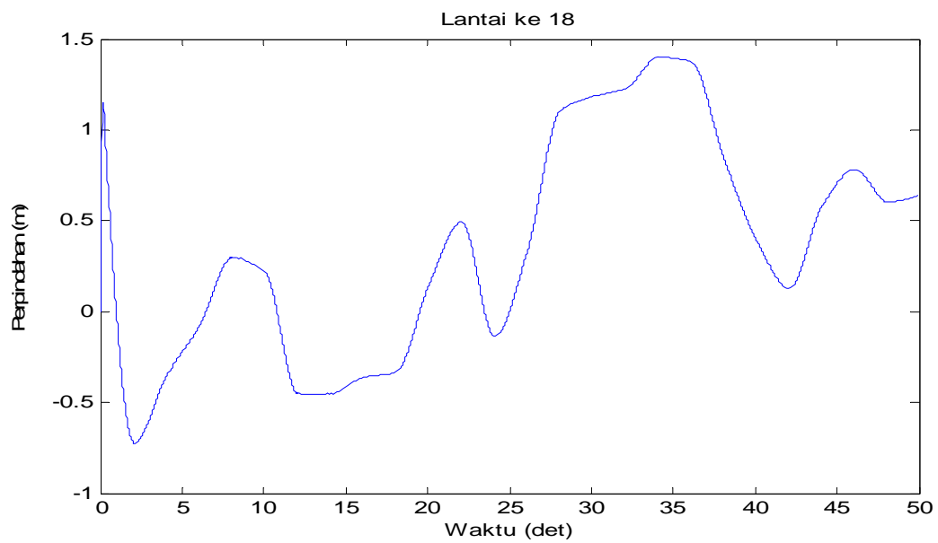
Gambar 4.89 Perpindahan di lantai 18 akibat beban gempa El-Centro dan Angin
