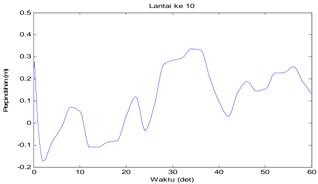
Gambar 4.101 Perpindahan di lantai 10 akibat beban gempa Flores dan Angin
