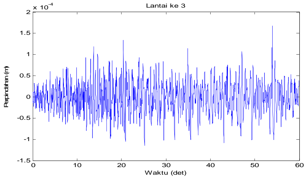
Gambar 4.34 Perpindahan di lantai 3 akibat beban gempa Flores
