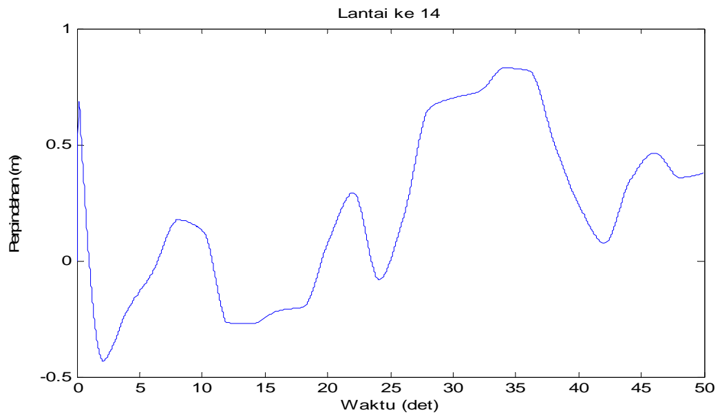
Gambar 4.85 Perpindahan di lantai 14 akibat beban gempa El-Centro dan Angin
