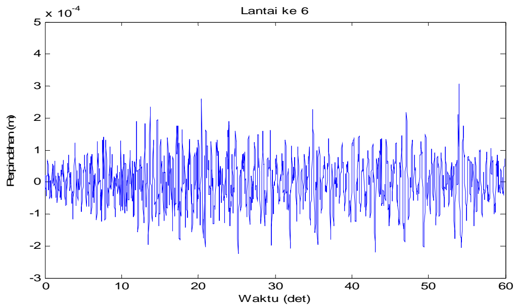
Gambar 4.37 Perpindahan di lantai 6 akibat beban gempa Flores
