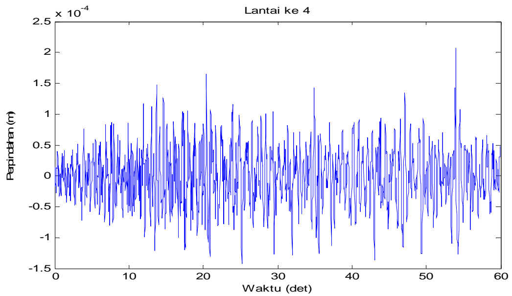
Gambar 4.35 Perpindahan di lantai 4 akibat beban gempa Flores
