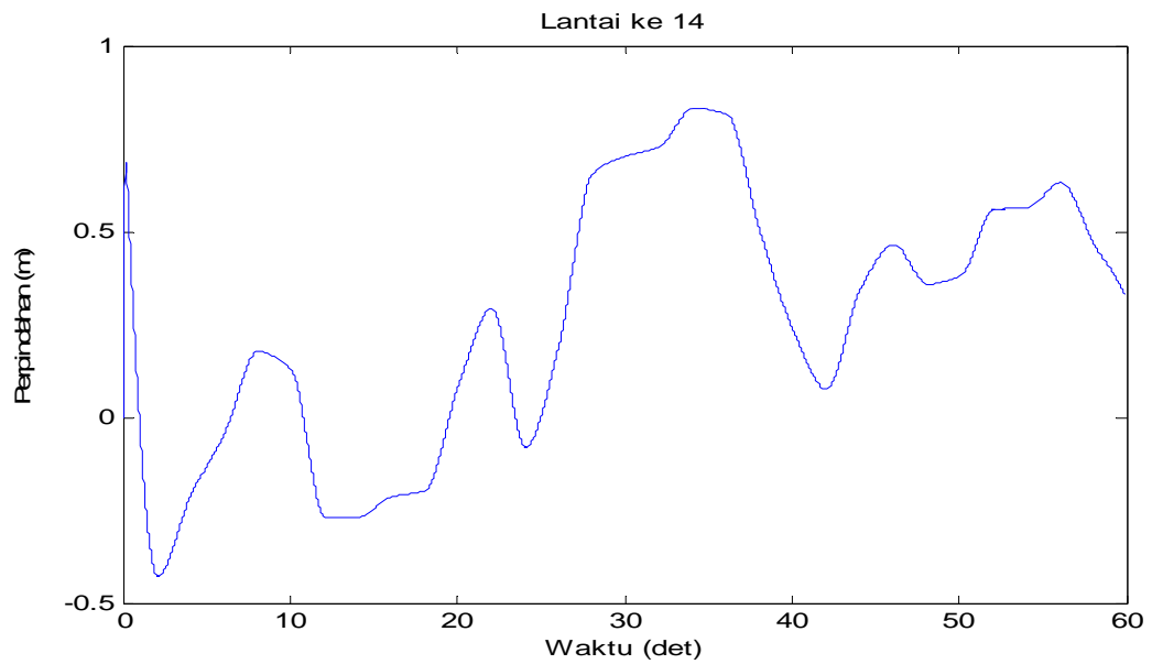
Gambar 4.105 Perpindahan di lantai 14 akibat beban gempa Flores dan Angin
