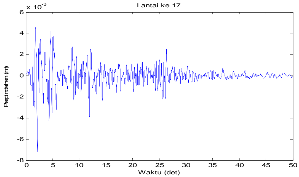
Gambar 4.28 Perpindahan di lantai 17 akibat beban gempa El-Centro
