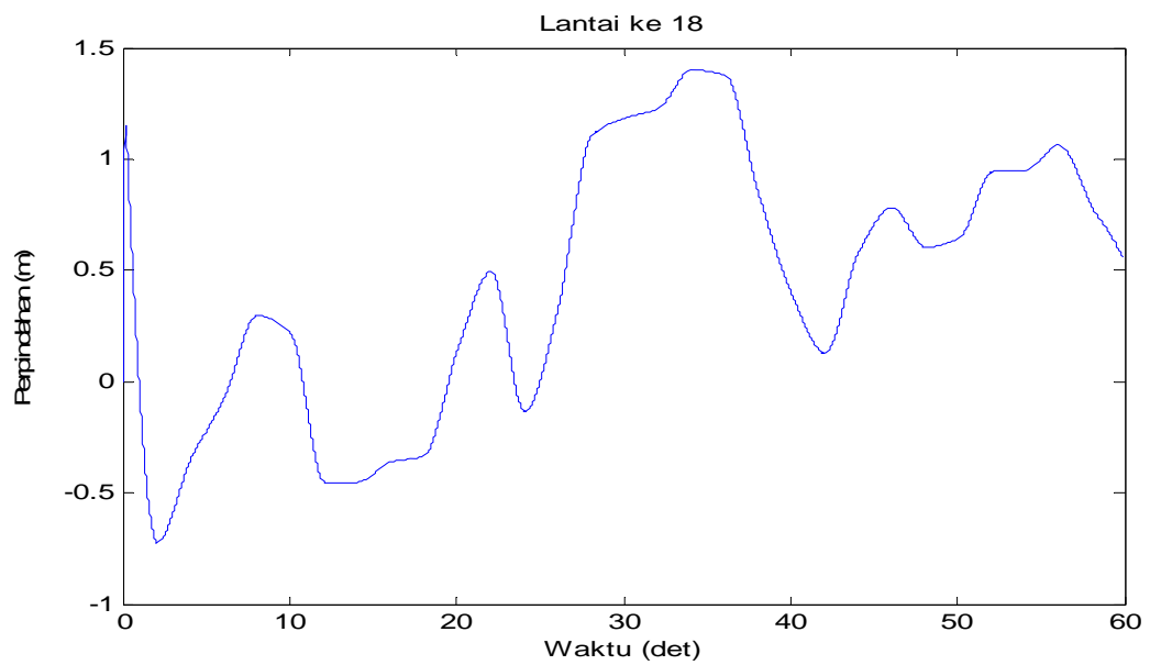
Gambar 4.69 Perpindahan di lantai 18 akibat beban Angin
