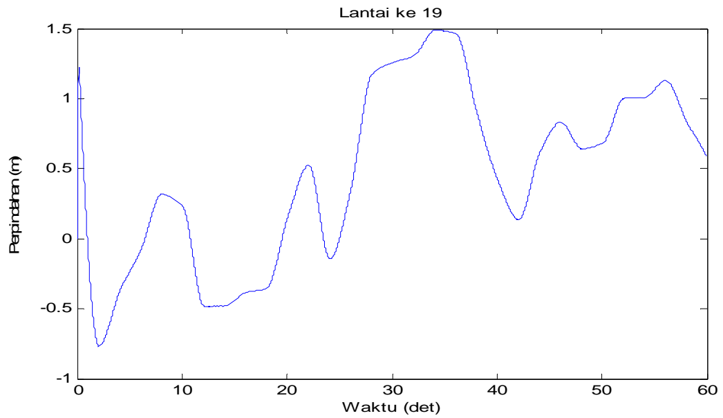
Gambar 4.110 Perpindahan di lantai 19 akibat beban gempa Flores dan Angin
