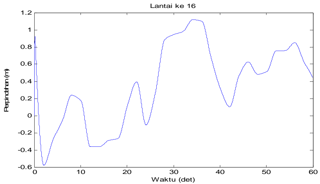
Gambar 4.67 Perpindahan di lantai 16 akibat beban Angin
