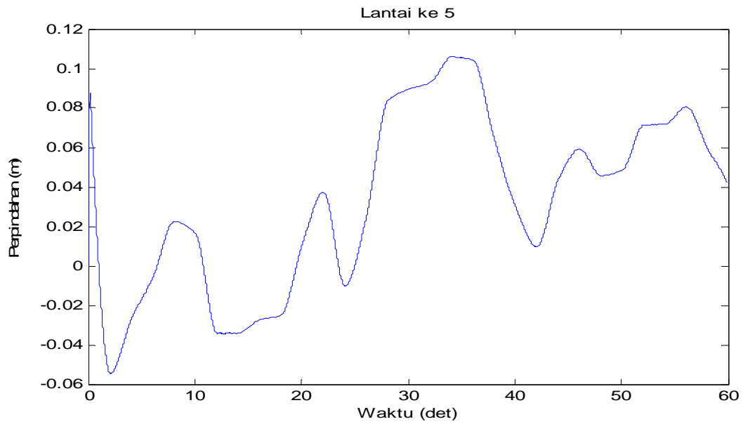
Gambar 4.96 Perpindahan di lantai 5 akibat beban gempa Flores dan Angin
