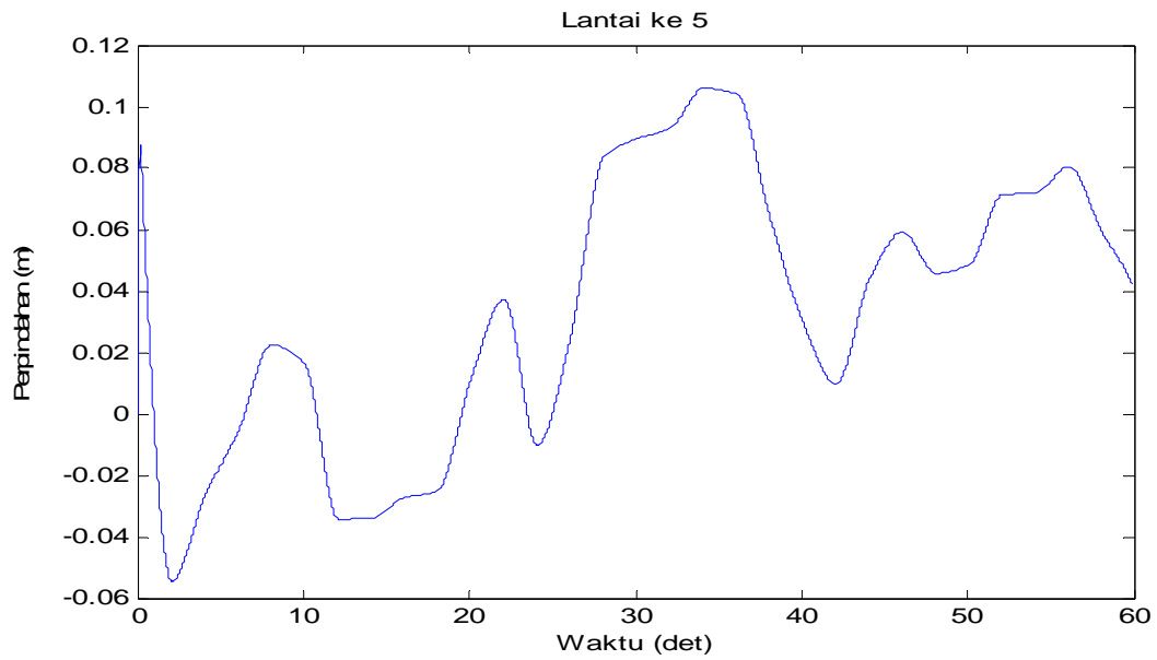
Gambar 4.56 Perpindahan di lantai 5 akibat beban Angin
