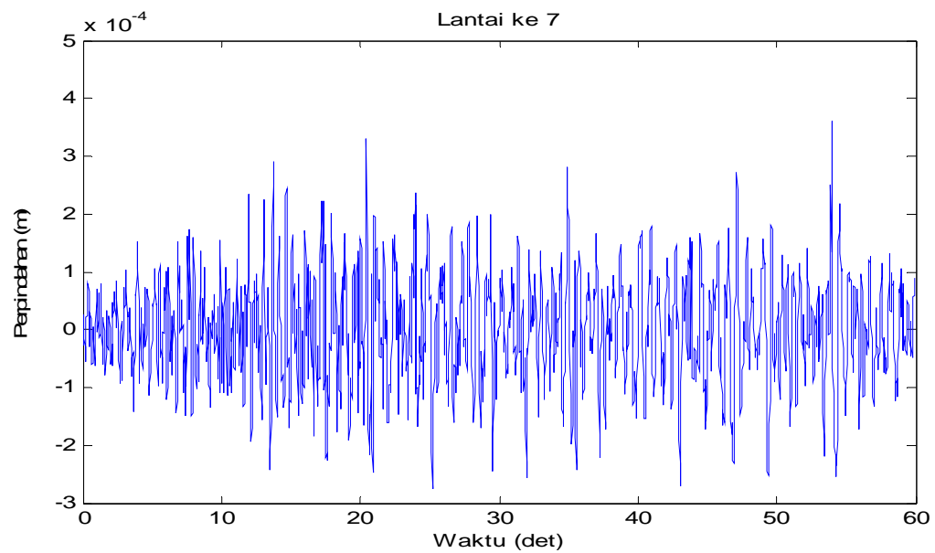
Gambar 4.38 Perpindahan di lantai 7 akibat beban gempa Flores
