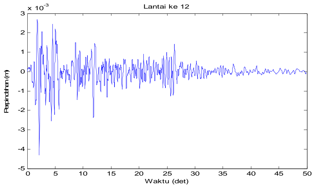
Gambar 4.23 Perpindahan di lantai 12 akibat beban gempa El-Centro
