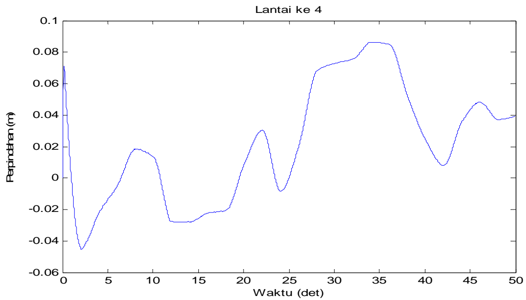
Gambar 4.75 Perpindahan di lantai 4 akibat beban gempa El-Centro dan Angin
