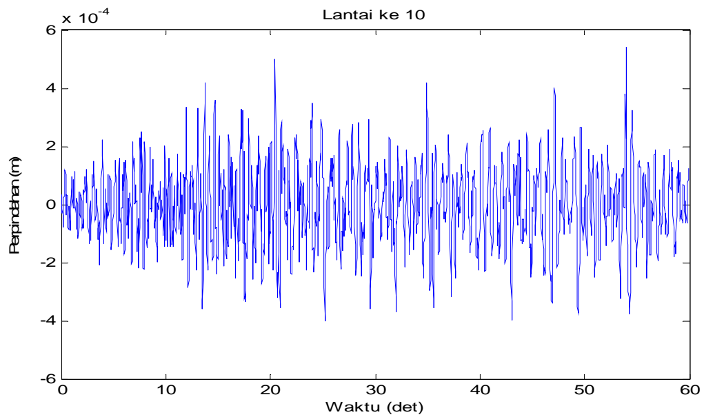
Gambar 4.41 Perpindahan di lantai 10 akibat beban gempa Flores
