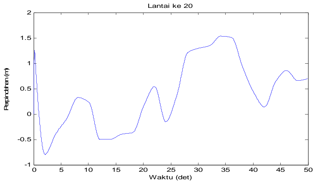
Gambar 4.91 Perpindahan di lantai 20 akibat beban gempa El-Centro dan Angin
