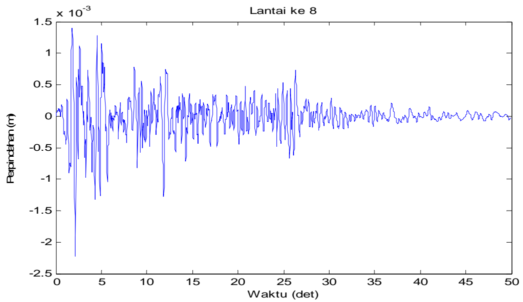
Gambar 4.19 Perpindahan di lantai 8 akibat beban gempa El-Centro
