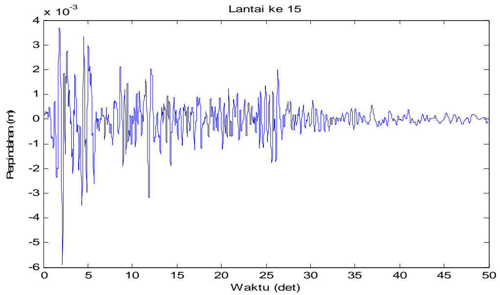
Gambar 4.26 Perpindahan di lantai 15 akibat beban gempa El-Centro
