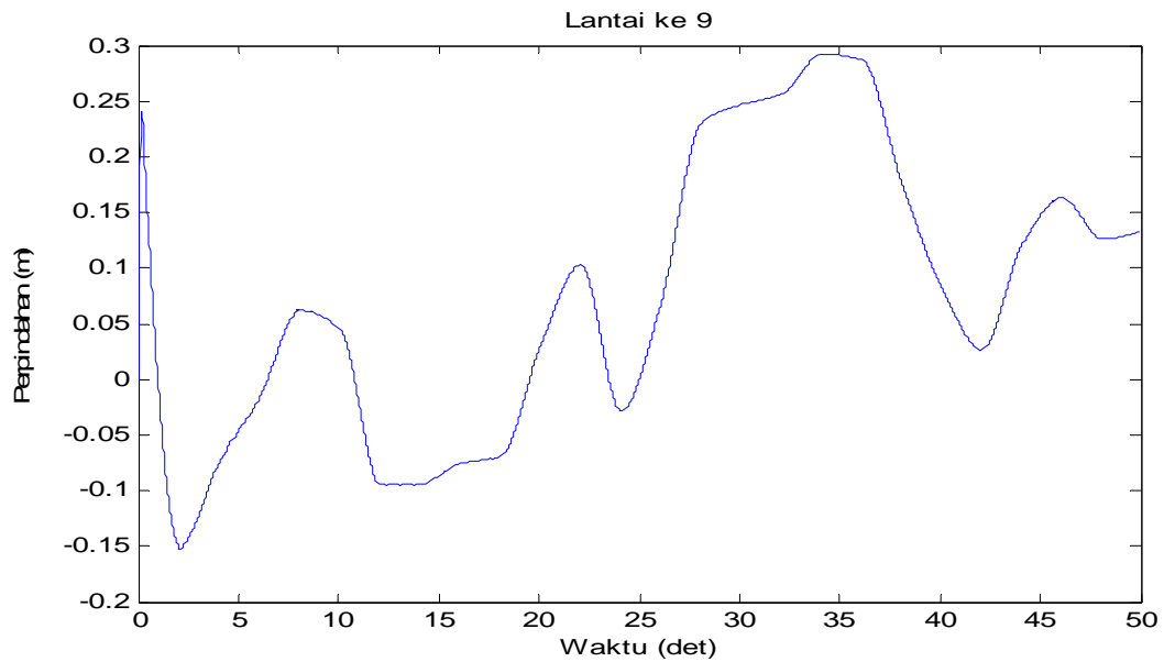
Gambar 4.80 Perpindahan di lantai 9 akibat beban gempa El-Centro dan Angin
