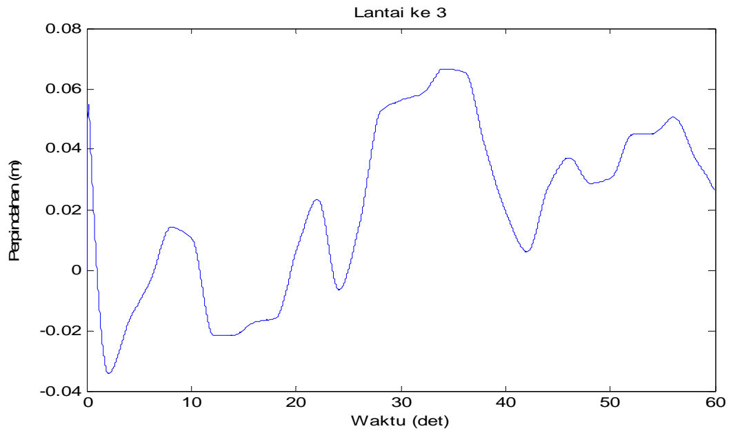
Gambar 4.94 Perpindahan di lantai 3 akibat beban gempa Flores dan Angin
