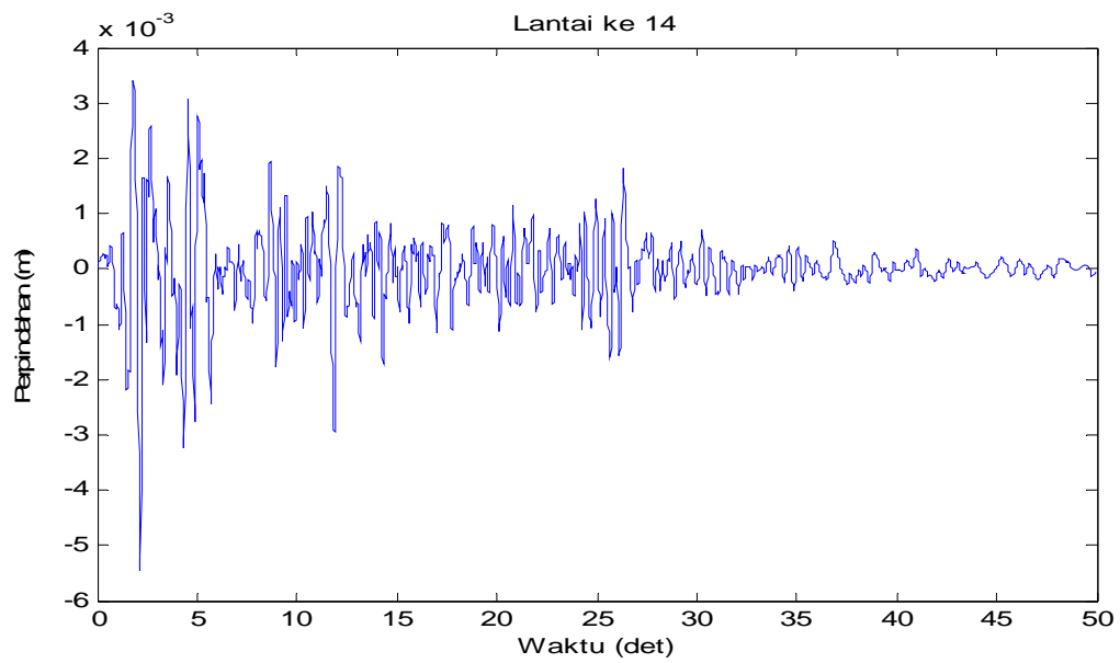
Gambar 4.25 Perpindahan di lantai 14 akibat beban gempa El-Centro
