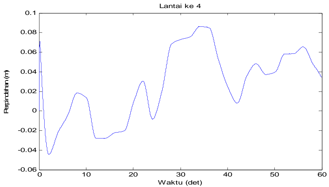
Gambar 4.95 Perpindahan di lantai 4 akibat beban gempa Flores dan Angin
