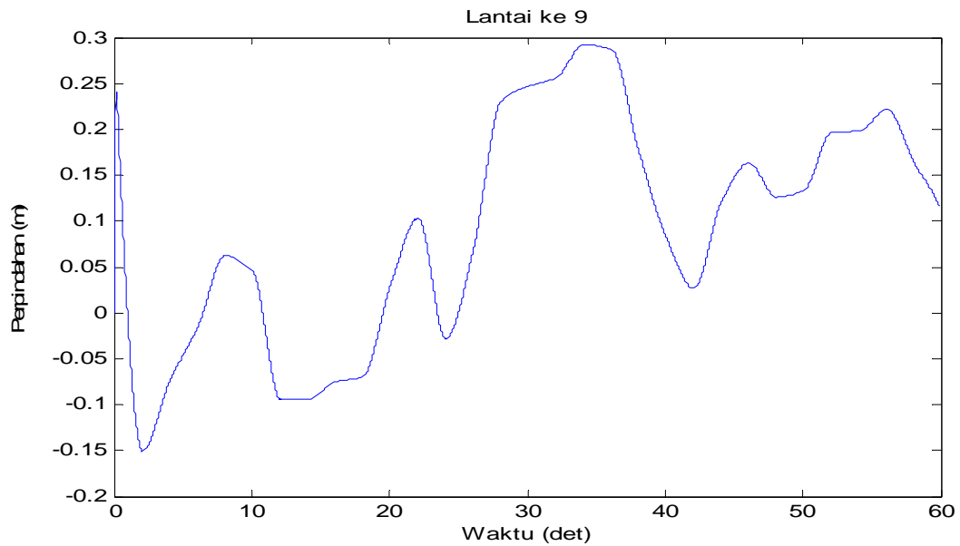
Gambar 4.100 Perpindahan di lantai 9 akibat beban gempa Flores dan Angin
