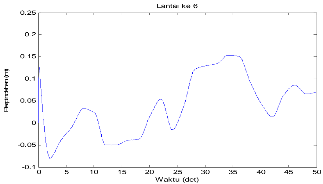
Gambar 4.77 Perpindahan di lantai 6 akibat beban gempa El-Centro dan Angin
