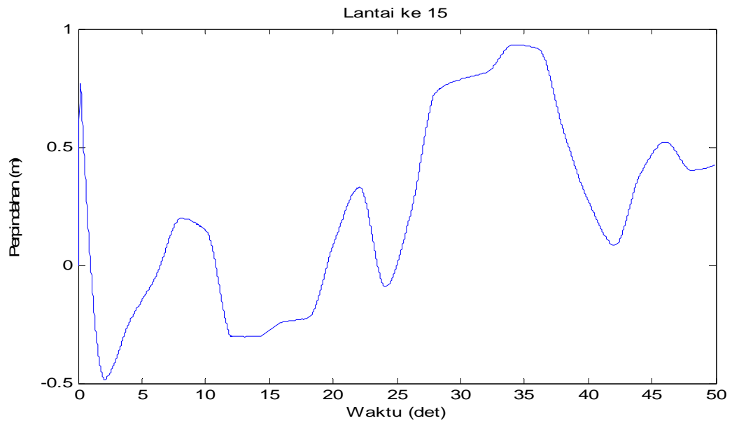
Gambar 4.86 Perpindahan di lantai 15 akibat beban gempa El-Centro dan Angin
