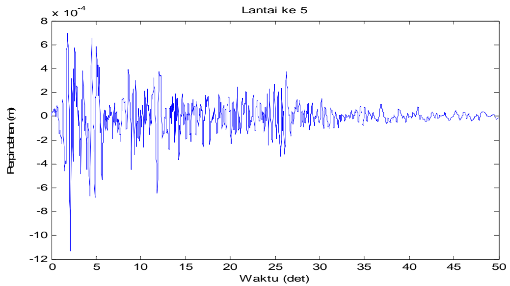
Gambar 4.16 Perpindahan di lantai 5 akibat beban gempa El-Centro
