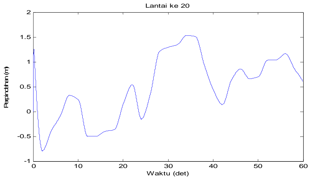
Gambar 4.111 Perpindahan di lantai 20 akibat beban gempa Flores dan Angin
