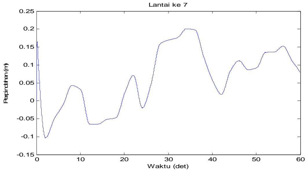
Gambar 4.58 Perpindahan di lantai 7 akibat beban Angin
