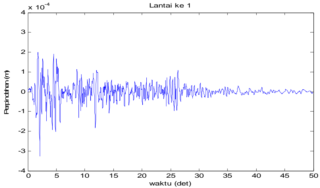
Gambar 4.12 Perpindahan di lantai 1 akibat beban gempa El-Centro
