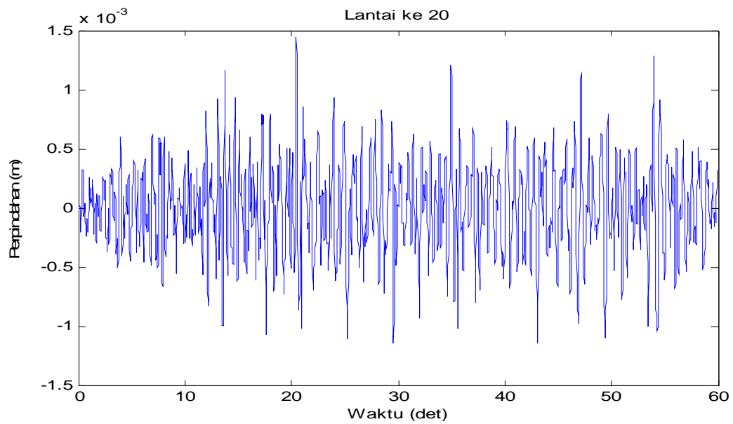
Gambar 4.51 Perpindahan di lantai 20 akibat beban gempa Flores
