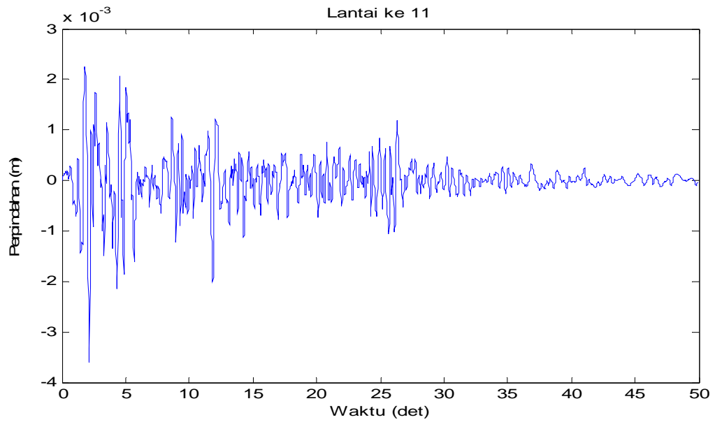
Gambar 4.22 Perpindahan di lantai 11 akibat beban gempa El-Centro
