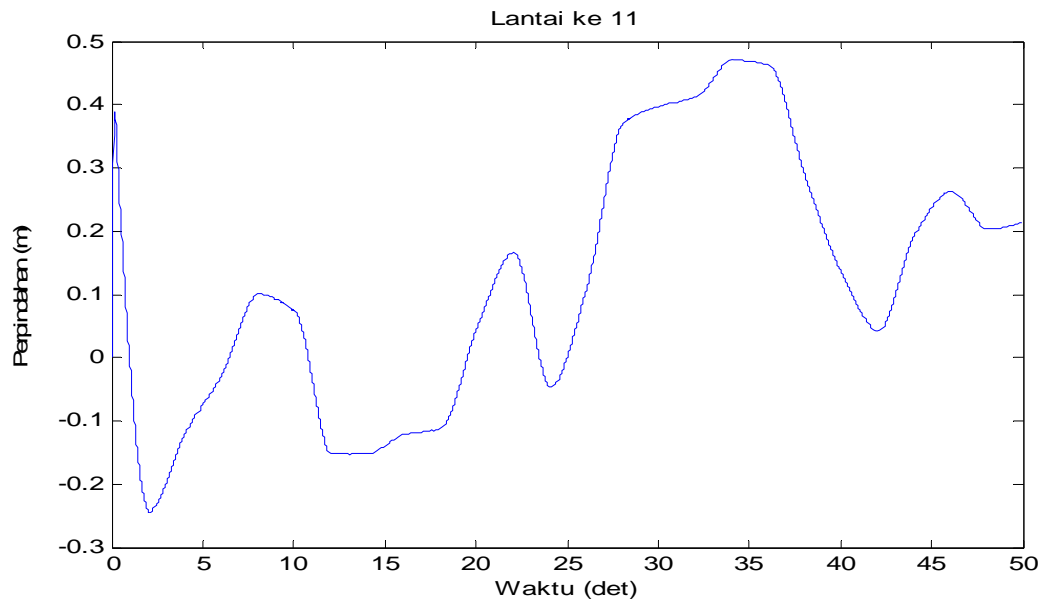
Gambar 4.82 Perpindahan di lantai 11 akibat beban gempa El-Centro dan Angin
