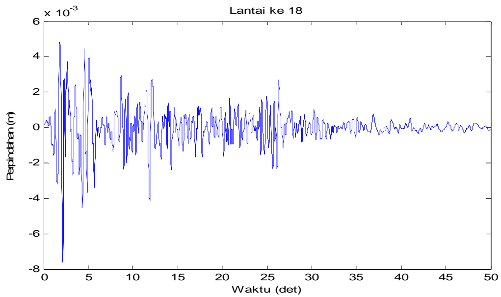
Gambar 4.29 Perpindahan di lantai 18 akibat beban gempa El-Centro
