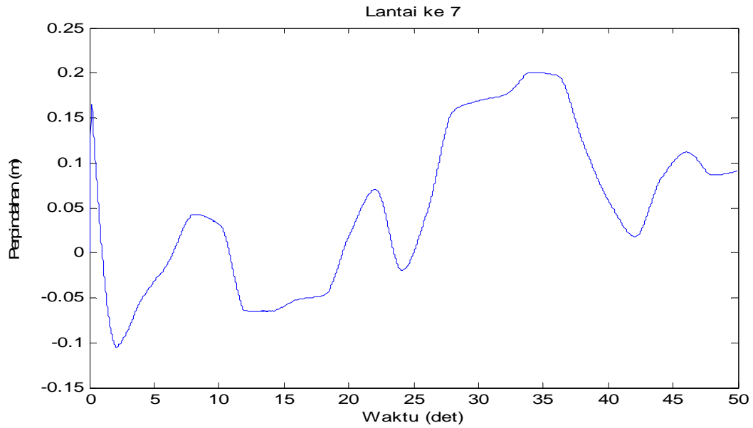
Gambar 4.78 Perpindahan di lantai 7 akibat beban gempa El-Centro dan Angin
