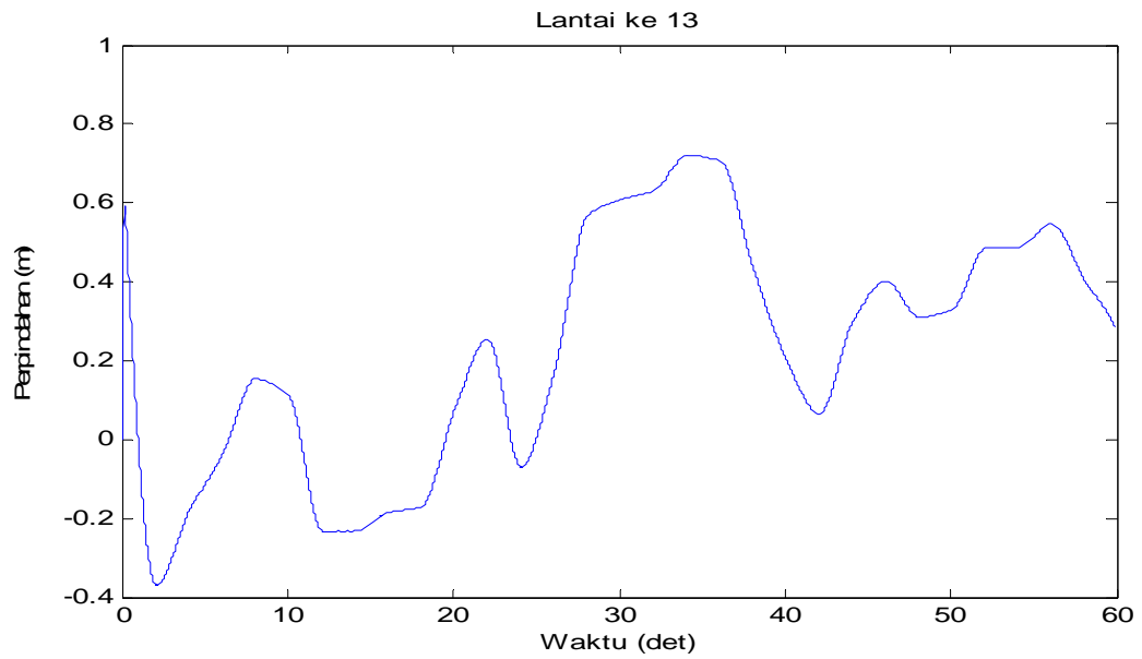
Gambar 4.104 Perpindahan di lantai 13 akibat beban gempa Flores dan Angin
