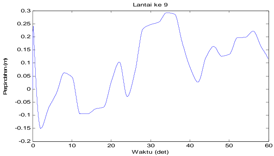
Gambar 4.60 Perpindahan di lantai 9 akibat beban Angin
