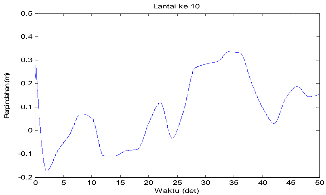
Gambar 4.81 Perpindahan di lantai 10 akibat beban gempa El-Centro dan Angin
