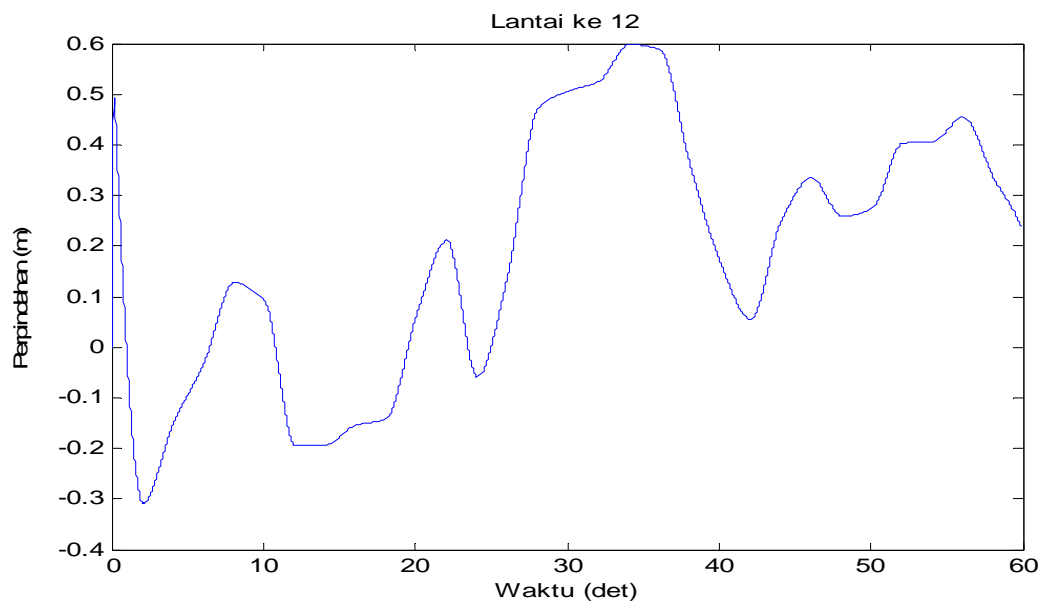
Gambar 4.63 Perpindahan di lantai 12 akibat beban Angin
