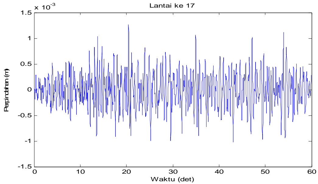
Gambar 4.48 Perpindahan di lantai 17 akibat beban gempa Flores
