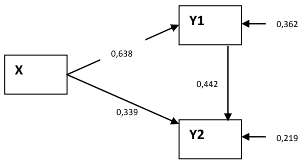
Gambar 5 Diagram Dekomposisi
