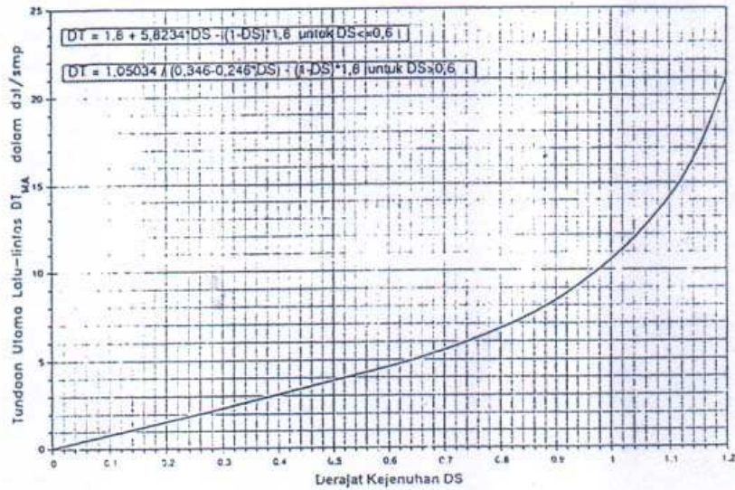
Grafik Hubungan Tundaan Lalu – Lintas Jalan Utama ( DTMA ) vs Derajat Kejenuhan
