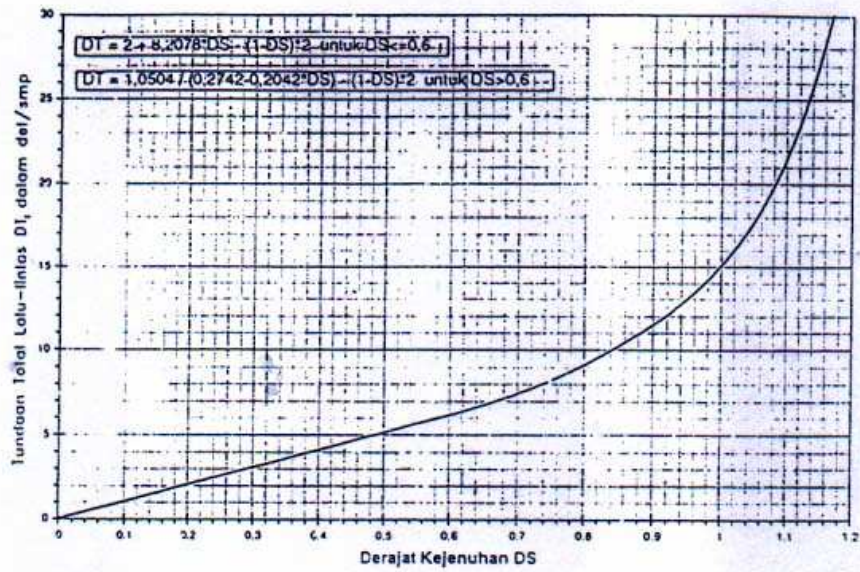
Grafik Hubungan Tundaan Lalu – Lintas Simpang ( DTI ) vs Derajat Kejenuhan
