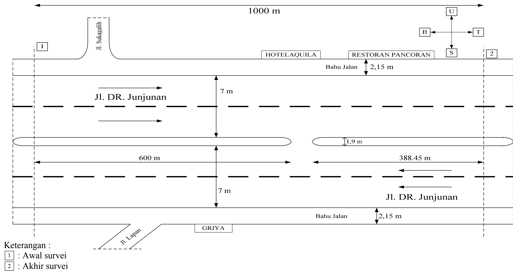
Gambar 3.3 Geometrik jalan
