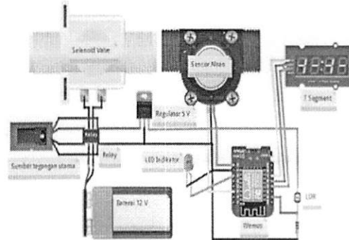
Gambar 9 Wiring Diagram Perangkat Water Meter
