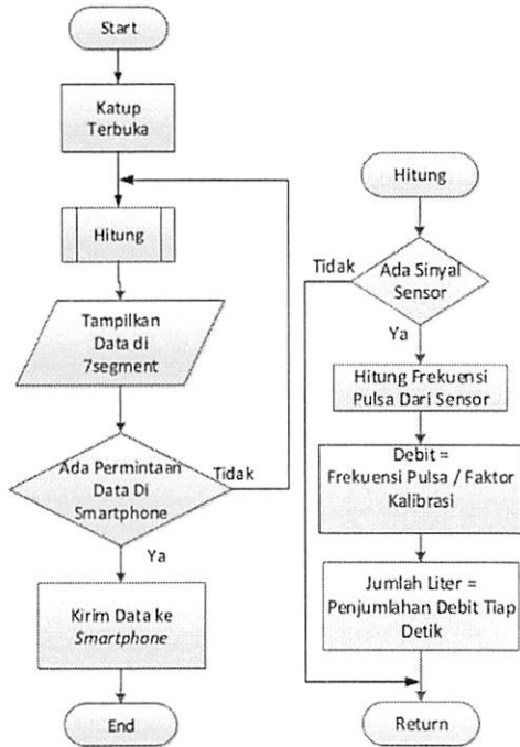
Gambar 10 Flowchart Program pada Perangkat Water Meter
