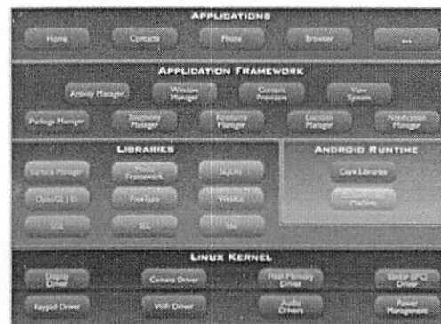
Gambar 6 Arsitektur Android
