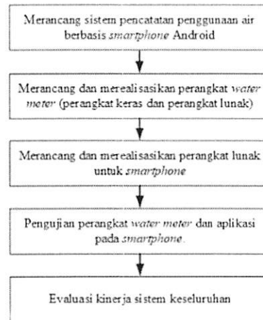
Gambar 7. Metodologi Penelitian
