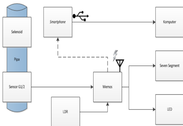
Gambar 8. Diagram Blok Sistem
