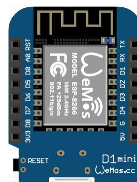
Gambar 3. Wemos D1 Mini
