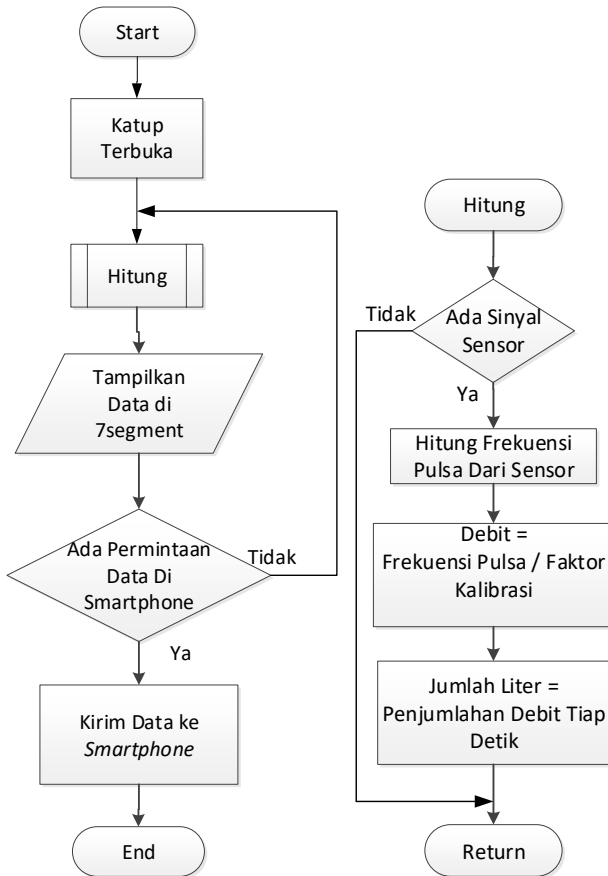
Gambar 10 Flowchart Program pada Perangkat Water Meter
