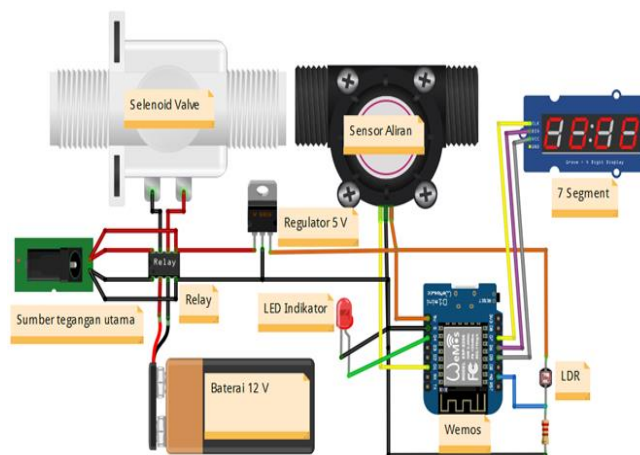
Gambar 9 Wiring Diagram Perangkat Water Meter
