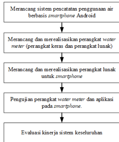
Gambar 7. Metodologi Penelitian
