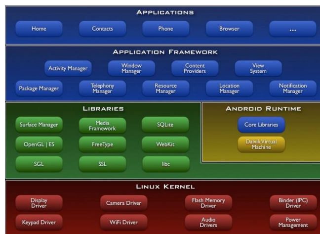
Gambar 6 Arsitektur Android
