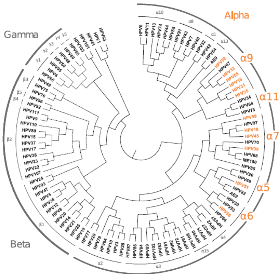
Gambar 6 Filogenetik HPV. 11
