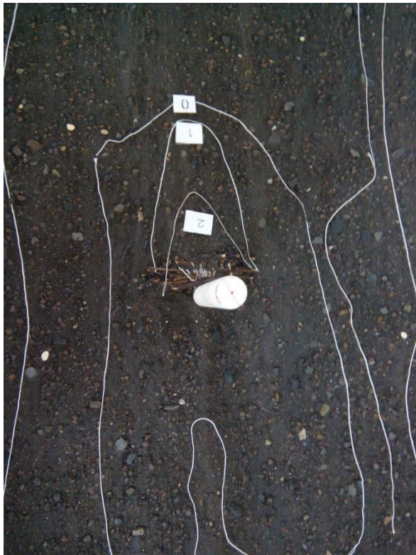
Gambar L.3.1 Pola Penggerusan Pilar Berbentuk Lingkaran Berdiameter 4cm dengan LWD Sejajar Sedimen
