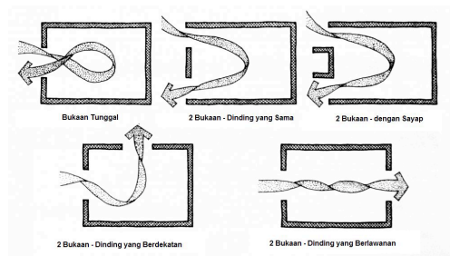
Gambar 2. Ragam Aliran Udara Berdasarkan Letak Bukaam Ruang Sumber: Sun, Wind & Light (2000)
