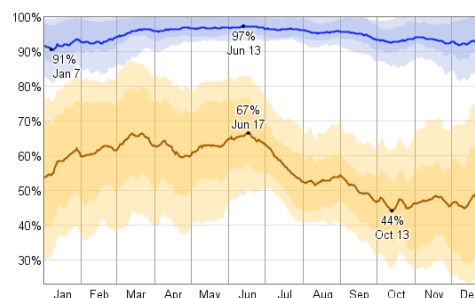
Gambar 11. Data Persentase Kelembaban di Kota Guilin tahun 2012
