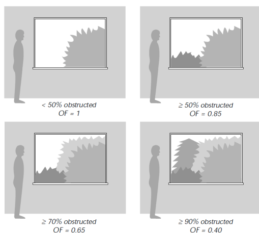
Gambar 9. Rasio Vegetasi pada Bukaam Sumber: Tips For Daylighting With Windows (1997)
