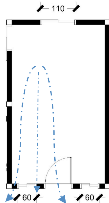
Gambar 22. Bukaannya Slider Sumber: Dokumentasi Pribadi
