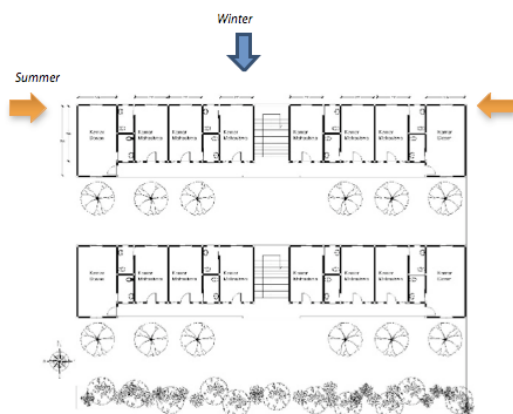
Gambar 14. Orientasi Bangunan Terhadap Sinar Matahari
