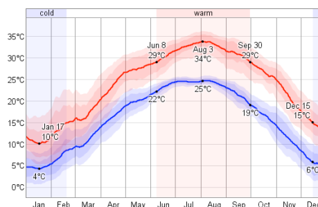
Gambar 10. Data Temperatur Udara di Kota Guilin tahun 2012
