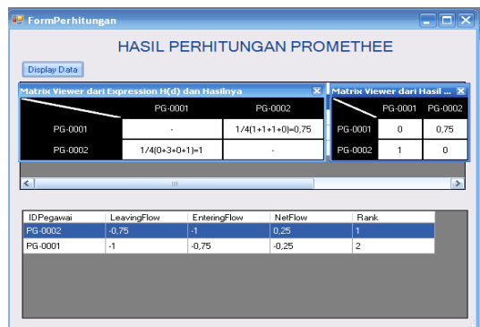
Gambar 5. Display Data
