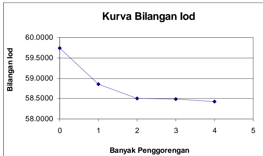
Gambar Kurva Bilangan Iod
